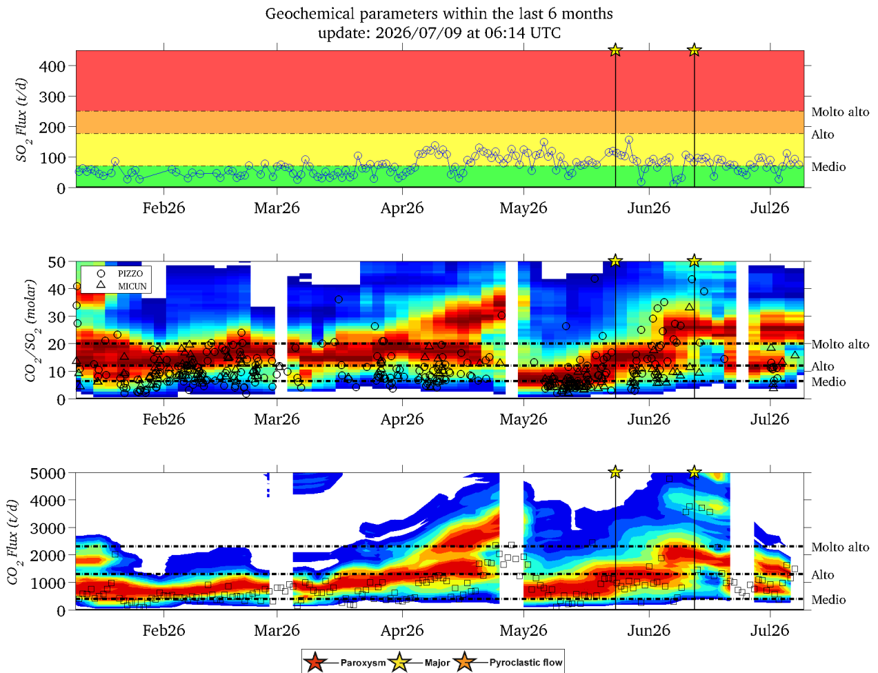
Figura 4 - Andamento dei parametri geochimici (flusso SO 2 e CO 2 e rapporto CO 2 /SO 2 ) negli ultimi 6 mesi (09 Gennaio – 09 Luglio 2026). Nei panelli CO 2 /SO 2 e flusso di CO 2 sono confrontati i risultati derivati attraverso due differenti metodi di processamento: (i) metodo tradizionale (punti e quadrati: basati sul valore medio del rapporto CO 2 /SO 2 in ogni finestra di acquisizione di 30 minuti; Aiuppa et al., 2009, JVGR) e (ii) nuovo metodo (Aiuppa et al., 2021, Sci Adv.) il cui output sono le distribuzioni di frequenza del rapporto e del flusso, rappresentate attraverso istogrammi di frequenza normalizzati (i colori rosso intenso rappresentano la mediana della distribuzione di frequenza). Si segnala che, a seguito dell'intervento di manutenzione della stazione Multi-GAS di Pizzo svolto in data 18 Giugno, le consuete procedure di verifica strumentale hanno permesso di riscontrare una inusuale degradazione nella calibrazione di uno dei sensori di misura, che ha richiesto il riprocessamento e ricalcolo dei rapporti C/S acquisiti nel periodo 22 Maggio – 18 Giugno 2026.
