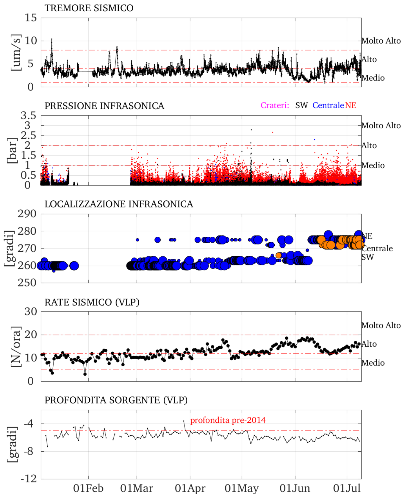
Figura 2 - Andamento dei parametri geofisici registrati a Stromboli nel periodo 09 Gennaio – 09 Luglio 2026.
