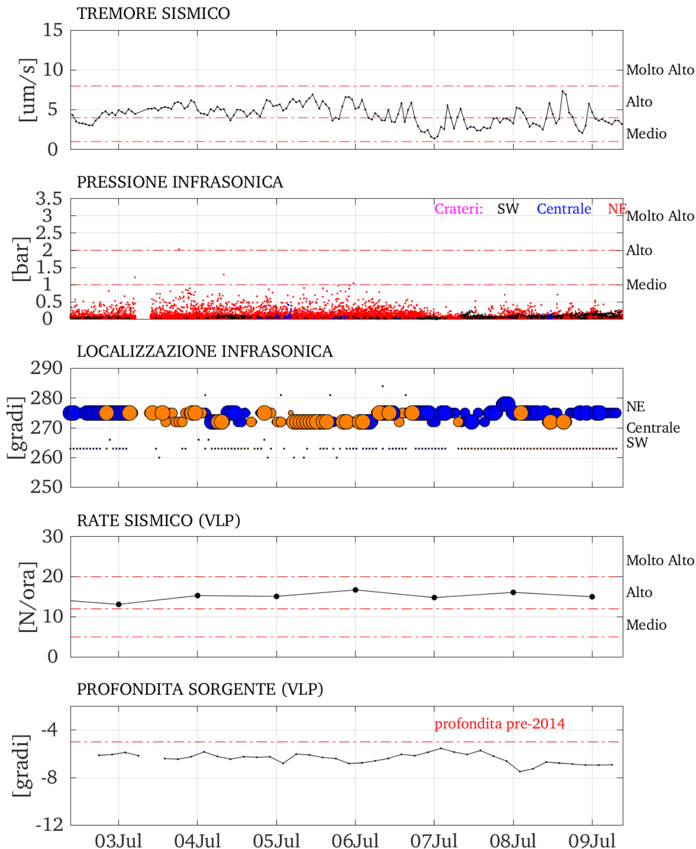
Figura 1 - Andamento dei parametri geofisici registrati a Stromboli nel periodo 03 Luglio – 09 Luglio 2026.
