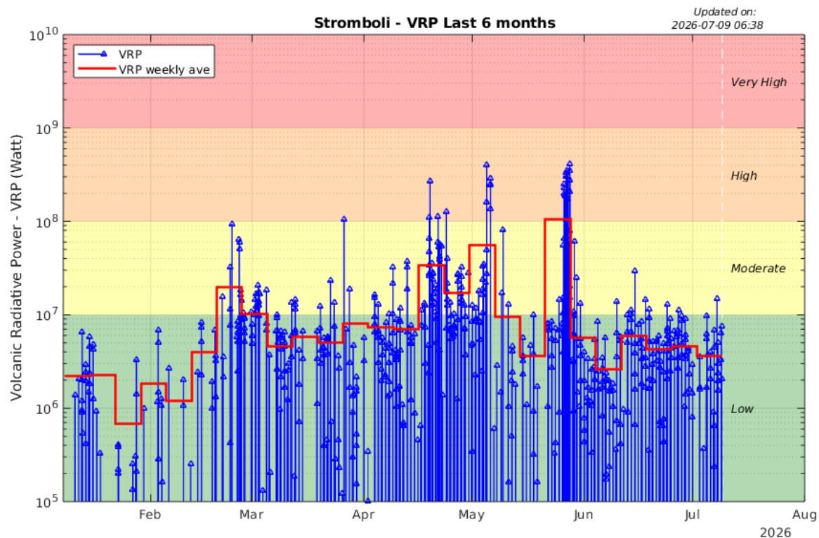
Figura 3 - Andamento del flusso termico (MODIS-VIIRS) nel periodo 09 Gennaio– 09 Luglio 2026.
