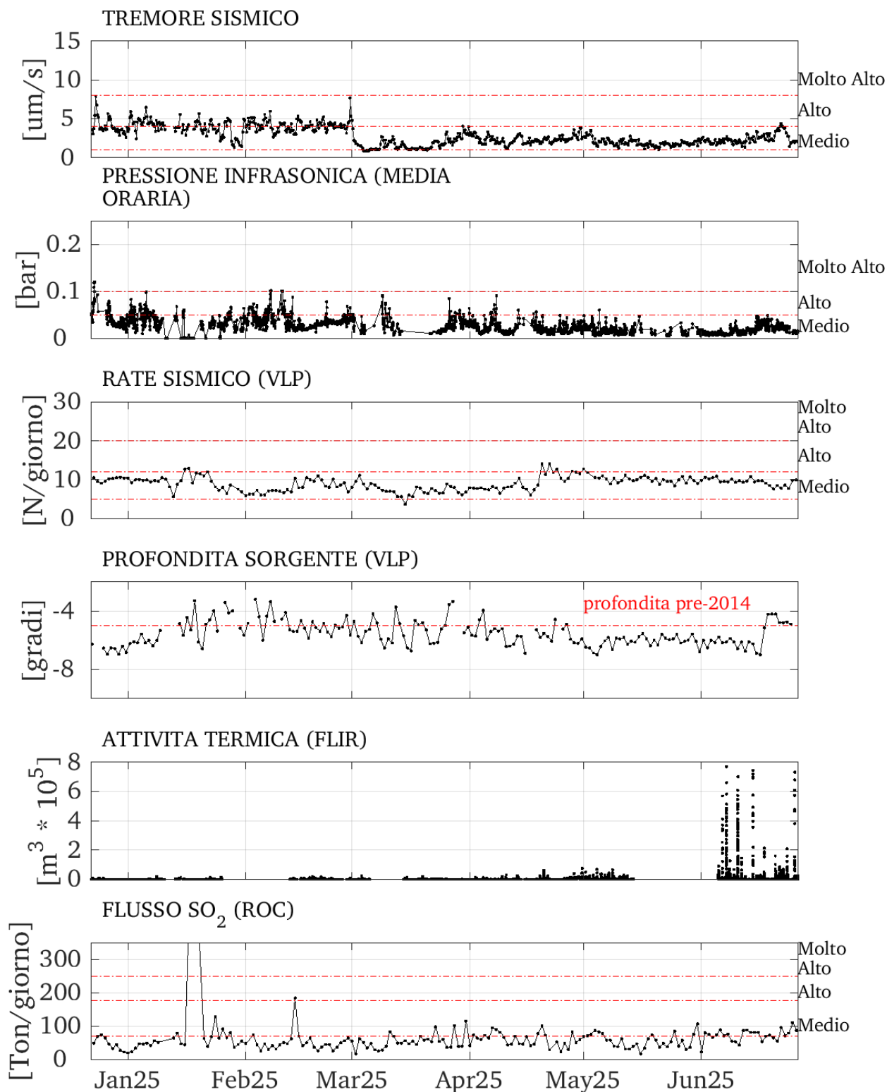
Figura 2 - Andamento dei parametri geofisici registrati a Stromboli nel periodo 26 dicembre 2024 – 26 giugno 2025.
