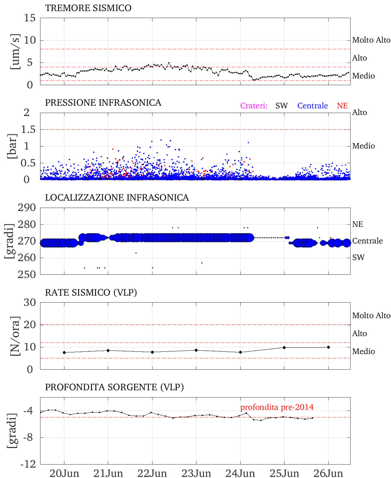
Figura 1 - Andamento dei parametri geofisici registrati a Stromboli nel periodo 20 giugno – 26 giugno 2025.
