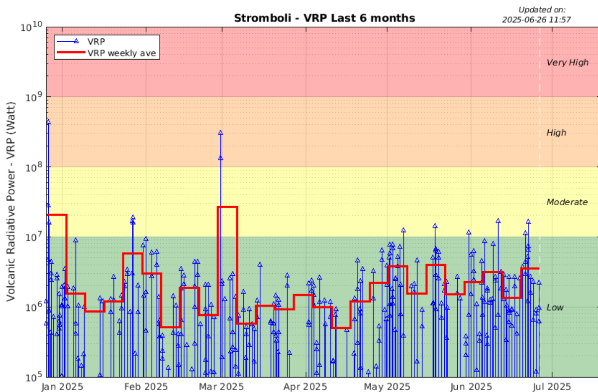
Figura 3 - Andamento del flusso termico (MODIS-VIIRS) nel periodo 26 dicembre 2024 – 26 giugno 2025.
