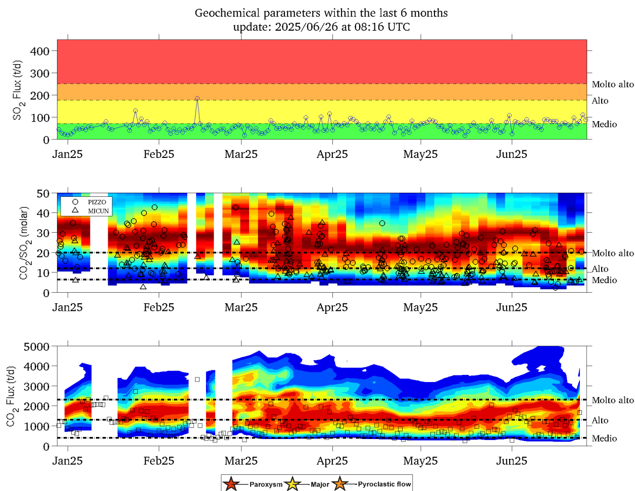
Figura 4 - Andamento dei parametri geochimici (flusso \text{SO}_2 e \text{CO}_2 e rapporto \text{CO}_2/\text{SO}_2 ) negli ultimi 6 mesi (26 dicembre 2024 – 26 giugno 2025). Nei pannelli \text{CO}_2/\text{SO}_2 e flusso di \text{CO}_2 sono confrontati i risultati derivati attraverso due differenti metodi di processamento: (i) metodo tradizionale (punti e quadrati: basati sul valore medio del rapporto \text{CO}_2/\text{SO}_2 in ogni finestra di acquisizione di 30 minuti; Aiuppa et al., 2009, JVGR) e (ii) nuovo metodo (Aiuppa et al., 2021, Sci Adv.) il cui output sono le distribuzioni di frequenza del rapporto e del flusso, rappresentate attraverso istogrammi di frequenza normalizzati (i colori rosso intenso rappresentano la mediana della distribuzione di frequenza).
