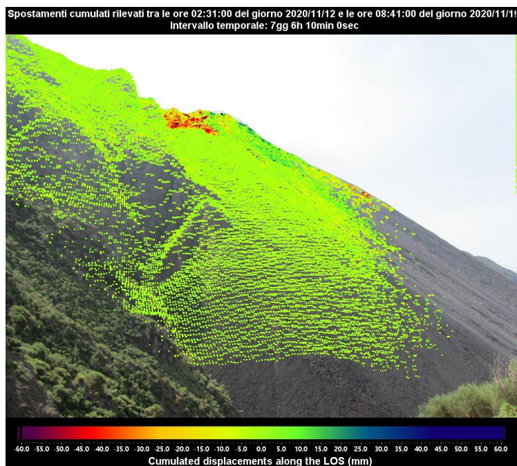
Figura 2 - Mappa degli spostamenti cumulati registrati dal sistema GB-InSAR NE400 riferito al tempo di 7 giorni e 6 ore, dalle ore 02:31 UTC (03:31 ore locali) del 12 novembre 2020 alle ore 08:41 UTC (09:41 ore locali) del 19 novembre 2020.
