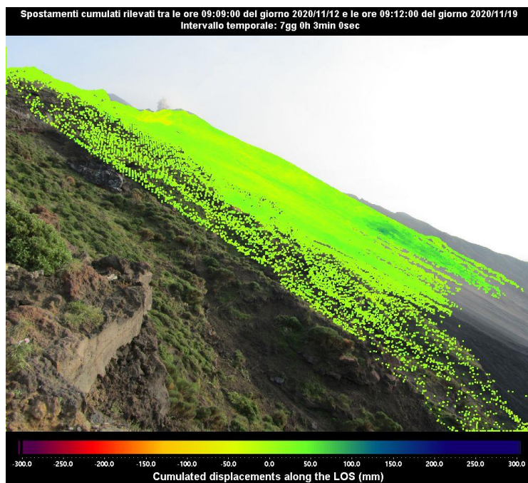
Figura 3 - Mappa degli spostamenti cumulati registrati dal sistema GB-InSAR NE190 riferito al tempo di 7 giorni, dalle ore 09:09 UTC (10:09 ore locali) del 12 novembre 2020 alle ore 09:12 UTC (10:12 ore locali) del 19 novembre 2020.
