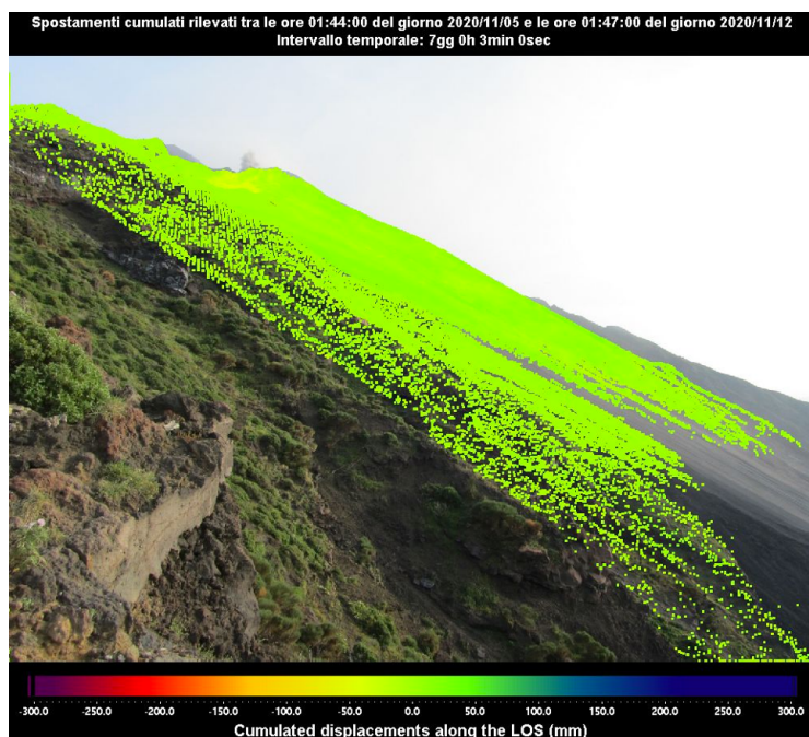
Figura 1 - Mappa degli spostamenti cumulati registrati dal sistema GB-InSAR NE190 riferito al tempo di 7 giorni 3 minuti, dalle ore 01:44 UTC (02:44 ore locali) del 5 novembre 2020 alle ore 01:47 UTC (02:47 ore locali) del 12 novembre 2020.
