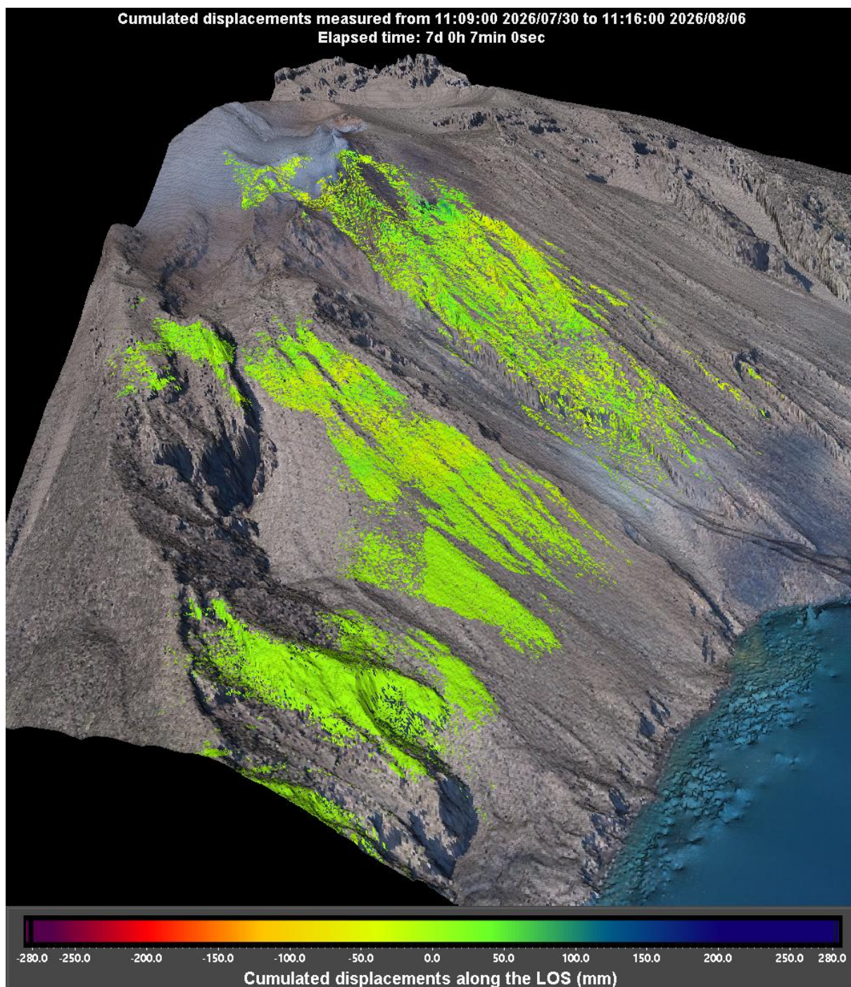
Figura 2 - Mappa cumulata degli spostamenti registrata dal sistema GBInSAR NE190 riferito al tempo di 7 giorni e 7 minuti dalle ore 11:09 UTC (13:09 ora locale) del 31 luglio 2026 alle ore 11:16 UTC (13:16 ora locale) del 06 agosto 2026.
