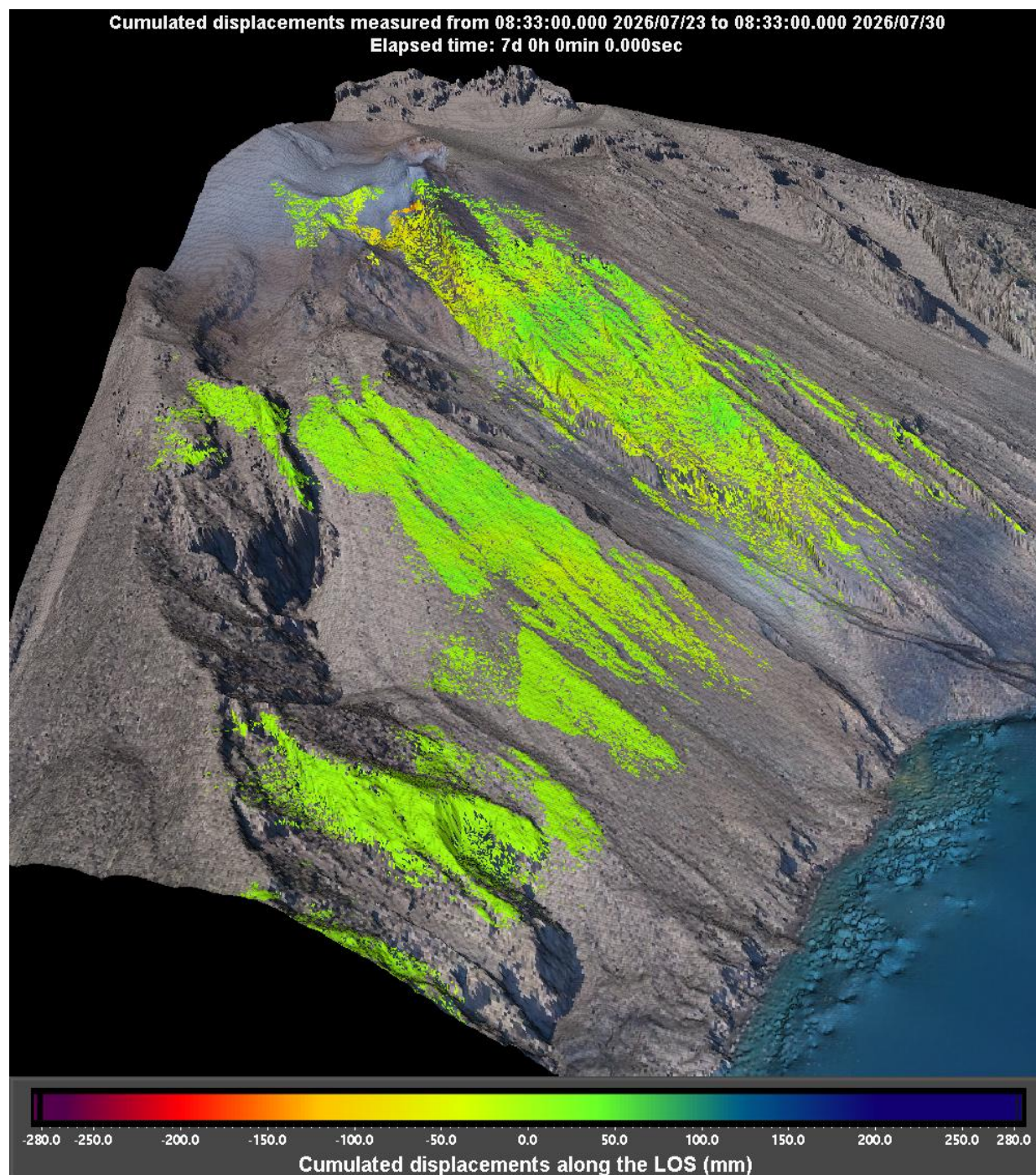
Figura 2 - Mappa cumulata degli spostamenti registrata dal sistema GBInSAR NE190 riferito al tempo di 7 giorni dalle ore 08:33 UTC (10:33 ora locale) del 23 luglio 2026 alle ore 08:33 UTC (10:33 ora locale) del 30 luglio 2026.
