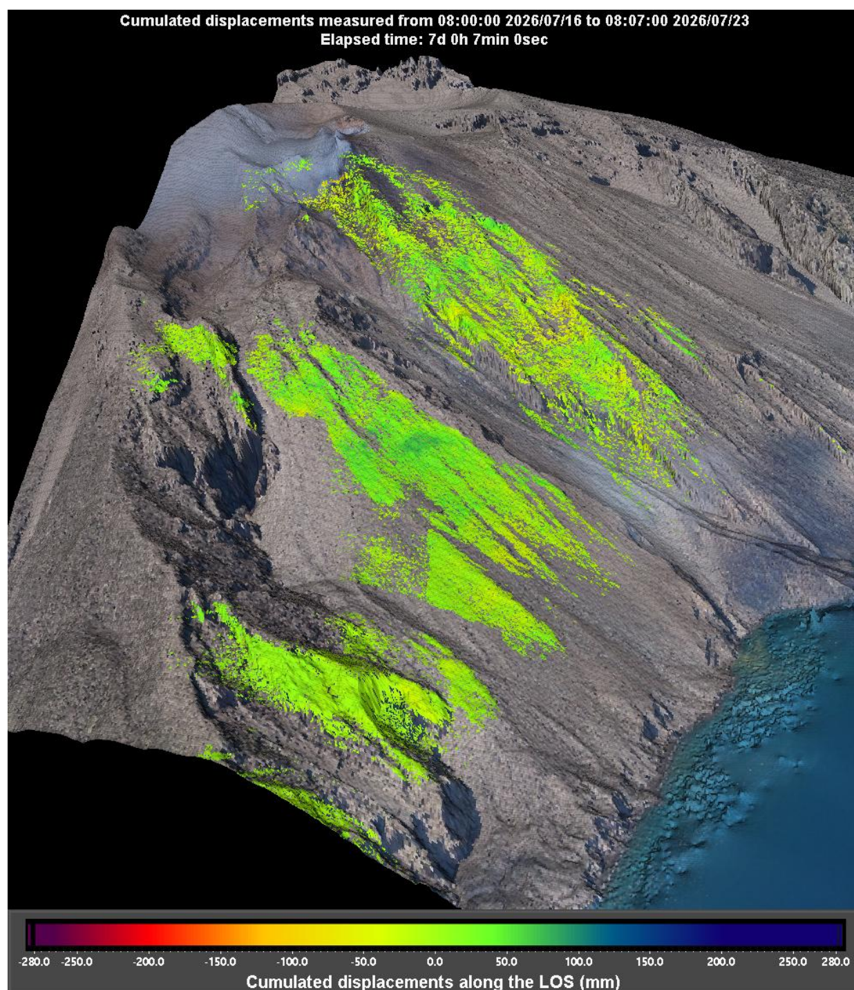
Figura 2 - Mappa cumulata degli spostamenti registrata dal sistema GBInSAR NE190 riferito al tempo di 7 giorni e 7 minuti dalle ore 08:00 UTC (10:00 ora locale) del 16 luglio 2026 alle ore 08:07 UTC (10:07 ora locale) del 23 luglio 2026.
