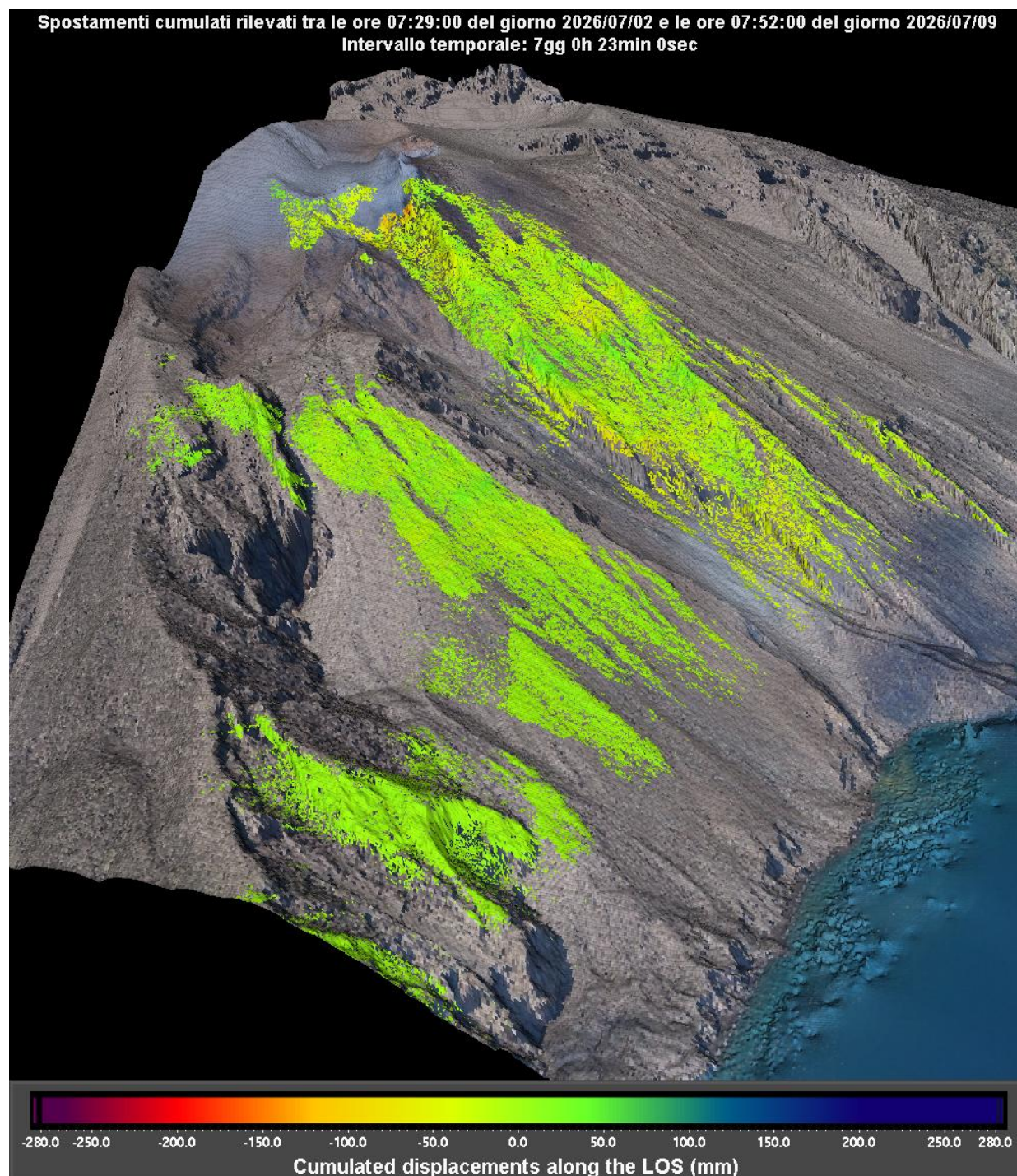
Figura 2 - Mappa cumulata degli spostamenti registrata dal sistema GBInSAR NE190 riferito al tempo di 7 giorni e 23 minuti dalle ore 07:29 UTC (09:29 ora locale) del 02 luglio 2026 alle ore 07:52 UTC (09:52 ora locale) del 09 luglio 2026.
