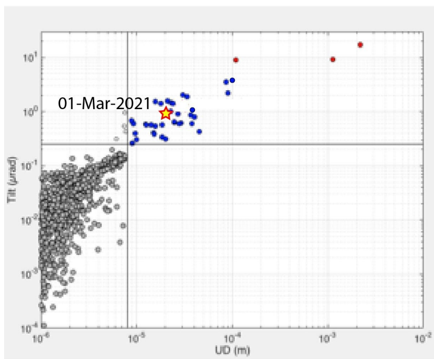
Figura 1. Il confronto tra le ampiezze sismica (UD) e la deformazione del suolo indicano che l'evento di oggi (stella) ricade nel campo delle esplosioni Maggiori.
