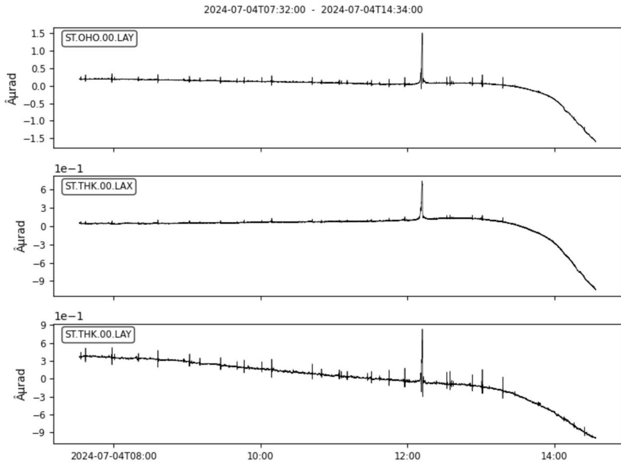
Figura 2 – Deformazione del suolo registrata dai tiltmetri.
