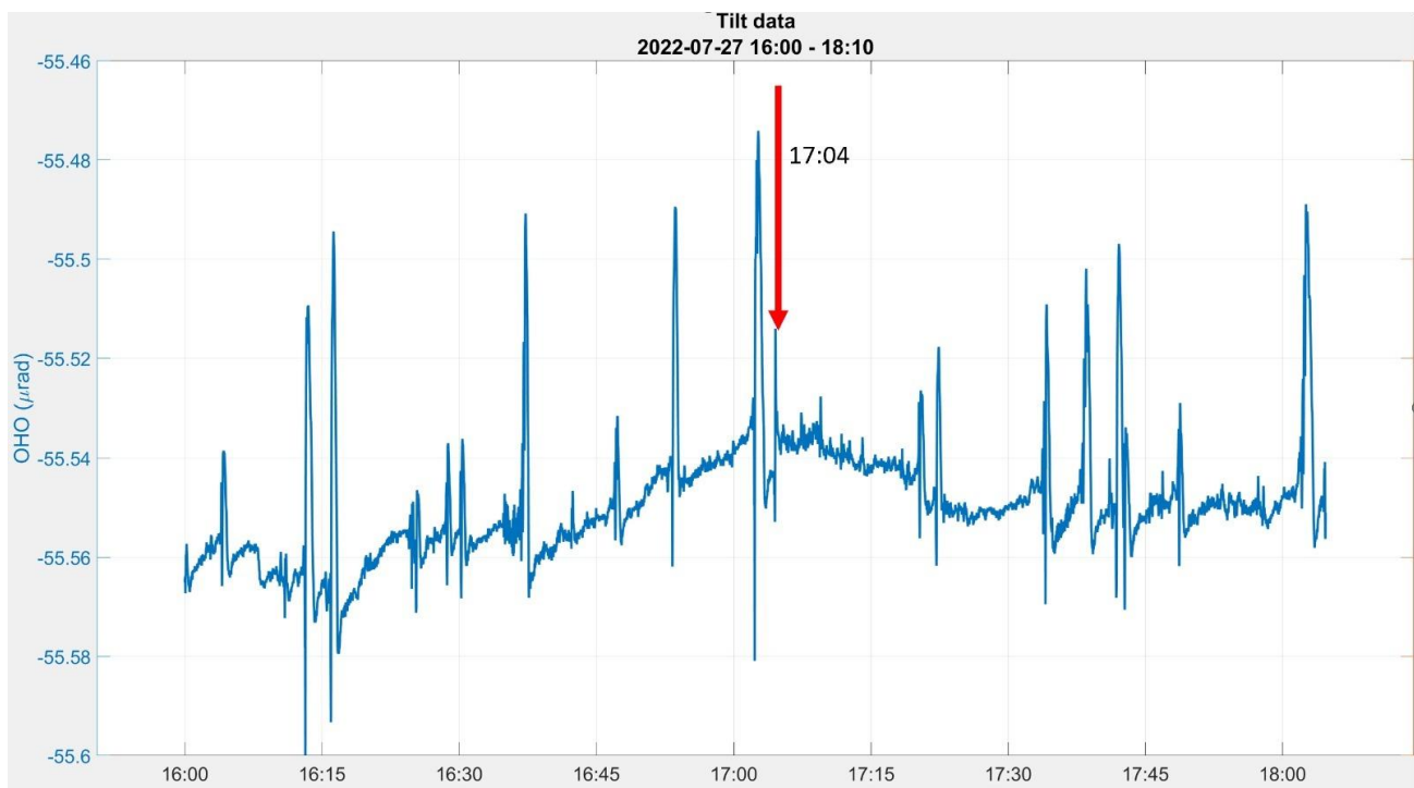
Figura 3 – Inflazione del suolo ( \mu\text{rad} ) registrata dal tiltmetro alla stazione OHO.
