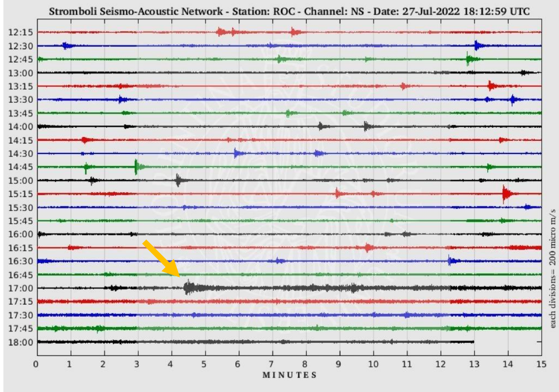
Fig. 2. Aumento del tremore sismico alla stazione ROC iniziato alle ore 17:04 UTC
