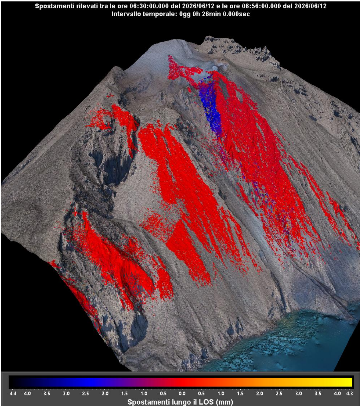
Figura 2 - Mappa cumulata degli spostamenti registrata dal sistema GBInSAR NE190 riferito al tempo di 26 minuti dalle ore 06:30 UTC (08:30 ora locale) alle ore 06:56 UTC (08:56 ora locale) del 12 giugno 2026.
