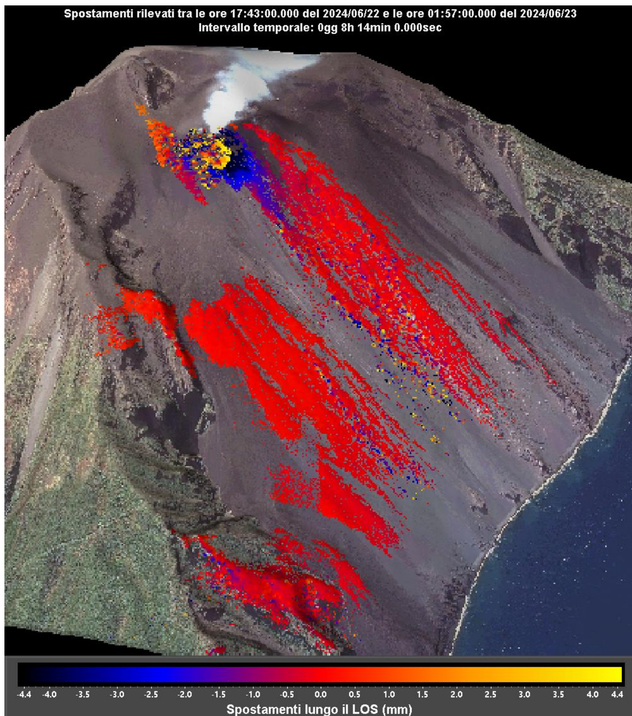
Figura 2 - Interferogramma registrato dal sistema GBInSAR NE190 riferita al tempo di 8 ore e 14 minuti dalle ore 17:43 UTC (19:43 ore locali) del 22 giugno 2024 alle ore 01:57 UTC (03:57 ore locali) del 23 gennaio 2024.
