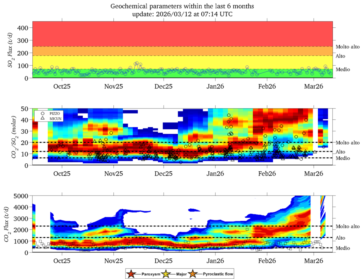
Figura 4 - Andamento dei parametri geochimici (flusso \text{SO}_2 e \text{CO}_2 e rapporto \text{CO}_2/\text{SO}_2 ) negli ultimi 6 mesi (12 Settembre 2025 – 12 Marzo 2026). Nei pannelli \text{CO}_2/\text{SO}_2 e flusso di \text{CO}_2 sono confrontati i risultati derivati attraverso due differenti metodi di processamento: (i) metodo tradizionale (punti e quadrati: basati sul valore medio del rapporto \text{CO}_2/\text{SO}_2 in ogni finestra di acquisizione di 30 minuti; Aiuppa et al., 2009, JVGR) e (ii) nuovo metodo (Aiuppa et al., 2021, Sci Adv.) il cui output sono le distribuzioni di frequenza del rapporto e del flusso, rappresentate attraverso istogrammi di frequenza normalizzati (i colori rosso intenso rappresentano la mediana della distribuzione di frequenza).
