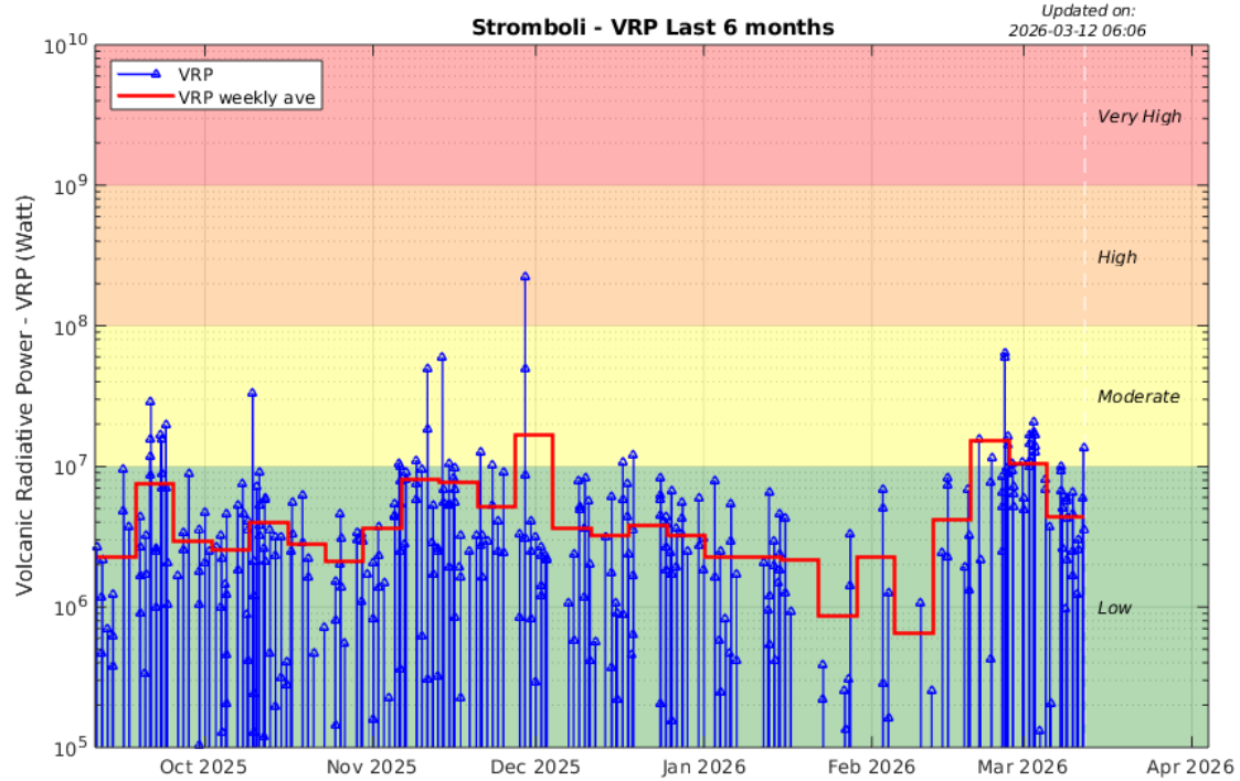
Figura 3 - Andamento del flusso termico (MODIS-VIIRS) nel periodo 12 Settembre 2025 – 12 Marzo 2026.
