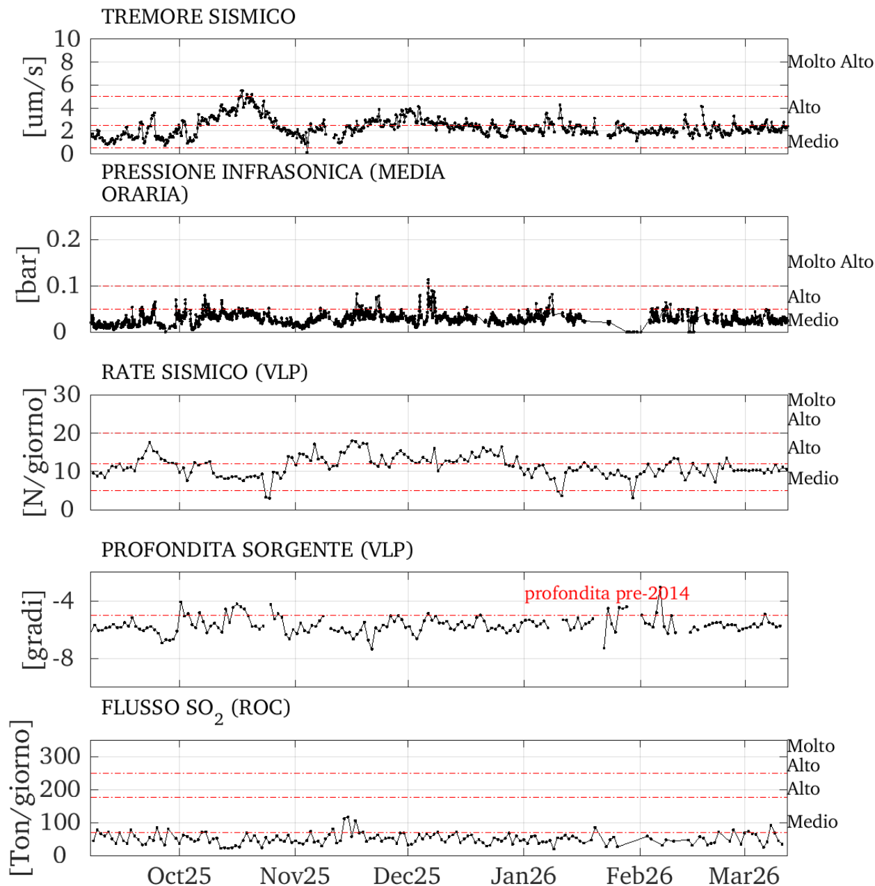
Figura 2 - Andamento dei parametri geofisici registrati a Stromboli nel periodo 12 Settembre 2025 – 12 Marzo 2026.
