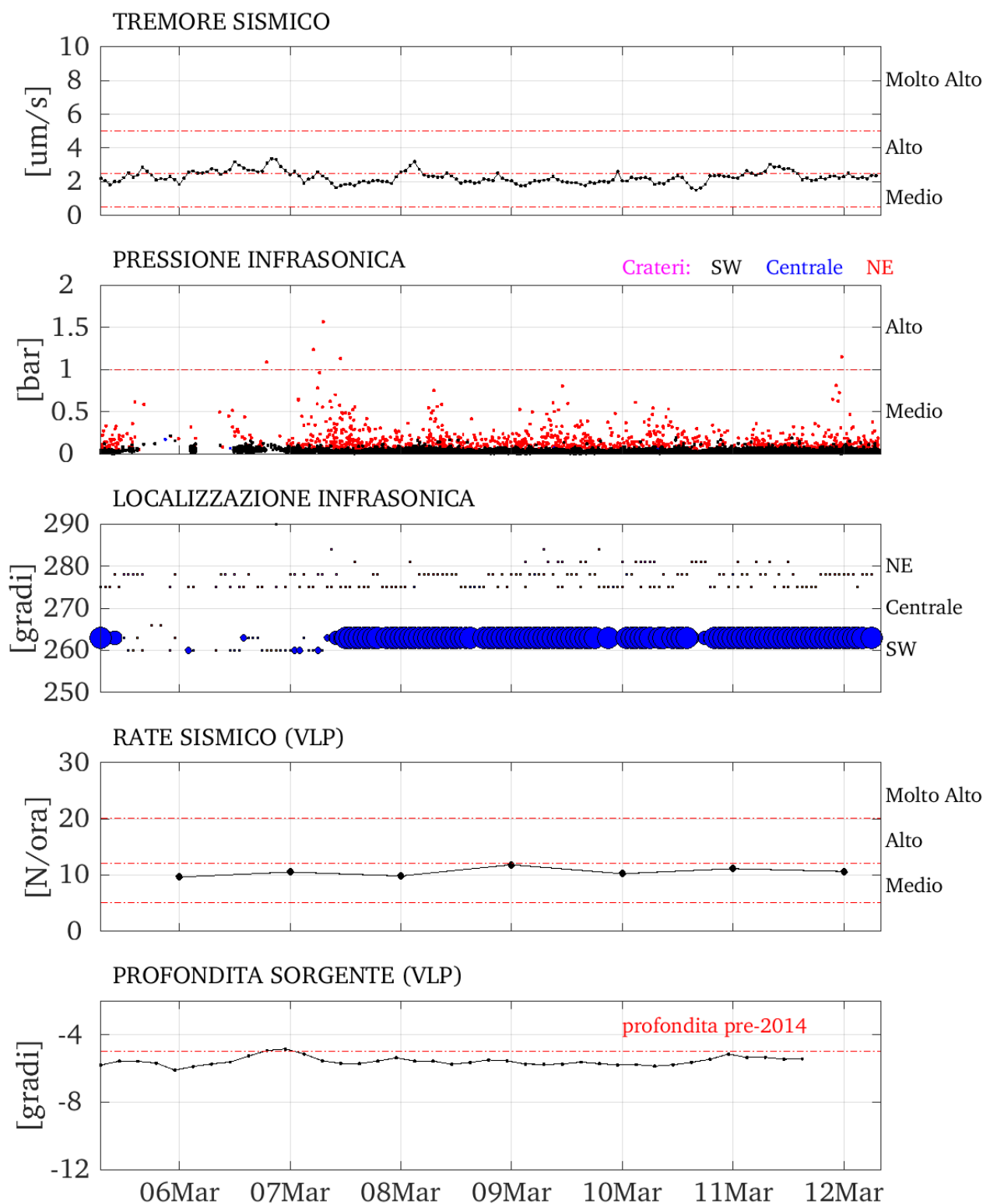
Figura 1 - Andamento dei parametri geofisici registrati a Stromboli nel periodo 06 Marzo – 12 Marzo 2026.
