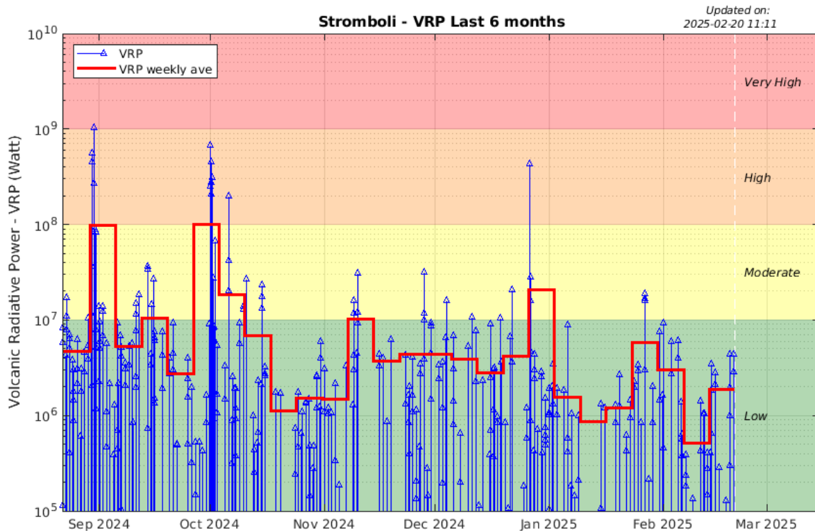
Figura 3 - Andamento del flusso termico (MODIS-VIIRS) nel periodo 20 Agosto 2024 – 20 Febbraio 2025.
