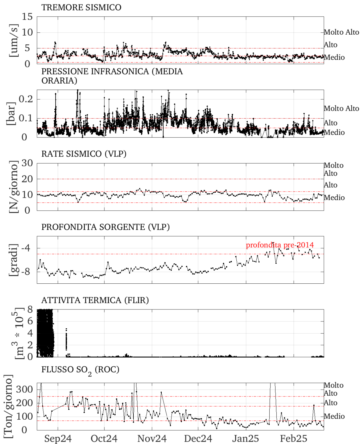
Figura 2 - Andamento dei parametri geofisici registrati a Stromboli nel periodo 20 Agosto 2024 – 20 Febbraio 2025.
