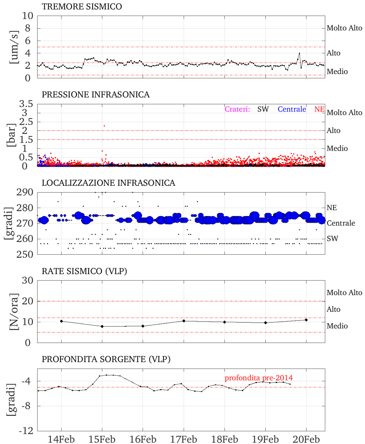
Figura 1 - Andamento dei parametri geofisici registrati a Stromboli nel periodo 14 Febbraio – 20 Febbraio 2025.
