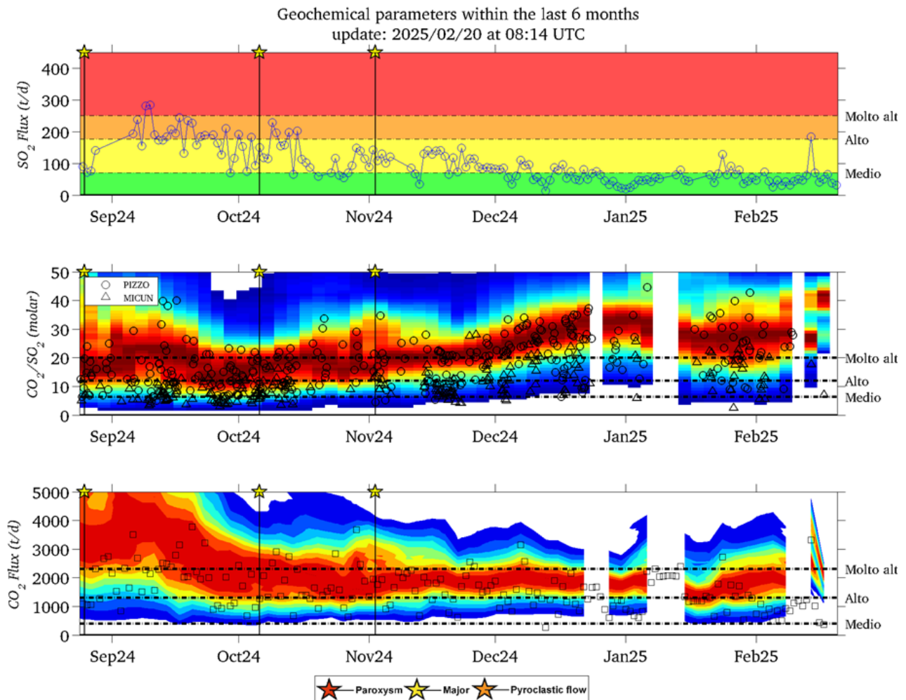
Figura 4 - Andamento dei parametri geochimici (flusso \text{SO}_2 e \text{CO}_2 e rapporto \text{CO}_2/\text{SO}_2 ) negli ultimi 6 mesi (20 Agosto 2024 – 20 Febbraio 2025). Nei pannelli \text{CO}_2/\text{SO}_2 e flusso di \text{CO}_2 sono confrontati i risultati derivati attraverso due differenti metodi di processamento: (i) metodo tradizionale (punti e quadrati: basati sul valore medio del rapporto \text{CO}_2/\text{SO}_2 in ogni finestra di acquisizione di 30 minuti; Aiuppa et al., 2009, JVGR ) e (ii) nuovo metodo (Aiuppa et al., 2021, Sci Adv. ) il cui output sono le distribuzioni di frequenza del rapporto e del flusso, rappresentate attraverso istogrammi di frequenza normalizzati (i colori rosso intenso rappresentano la mediana della distribuzione di frequenza).
