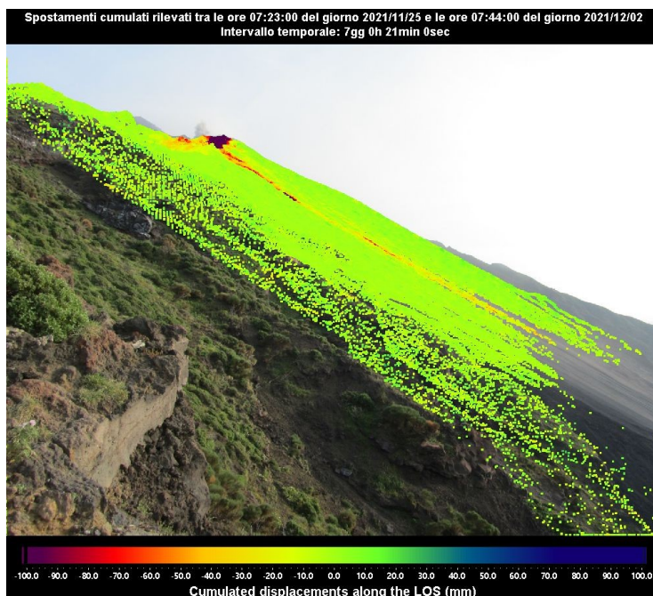
Figura 3 - Mappa degli spostamenti cumulati registrata dal sistema GB-InSAR NE190 riferita al tempo di 7 giorni e 21 minuti dalle ore 07:23 UTC (08:23 ore locali) del 25 novembre 2021 alle ore 07:44 UTC (08:44 ore locali) del 2 dicembre 2021.
