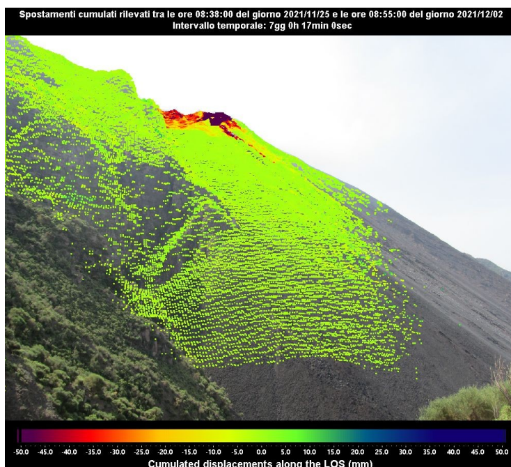
Figura 2 - Mappa degli spostamenti cumulati registrata dal sistema GB-InSAR NE400 riferita al tempo di 7 giorni e 17 minuti dalle ore 08:38 UTC (09:38 ore locali) del 25 novembre 2021 alle ore 08:55 UTC (09:55 ore locali) del 2 dicembre 2021.
