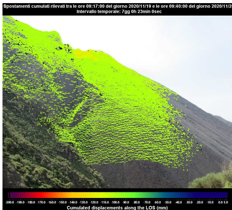
Figura 2 - Mappa degli spostamenti cumulati registrati dal sistema GB-InSAR NE400 riferito al tempo di 7 giorni e 23 ore, dalle ore 09:17 UTC (10:17 ore locali) del 19 novembre 2020 alle ore 09:40 UTC (10:40 ore locali) del 26 novembre 2020.
