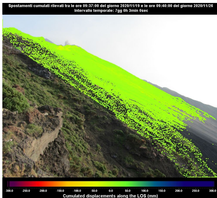
Figura 3 - Mappa degli spostamenti cumulati registrati dal sistema GB-InSAR NE190 riferito al tempo di 7 giorni e 3 minuti, dalle ore 09:37 UTC (10:37 ore locali) del 19 novembre 2020 alle ore 09:40 UTC (10:40 ore locali) del 26 novembre 2020.
