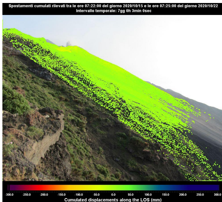
Figura 1 - Mappa degli spostamenti cumulati registrati dal sistema GB-InSAR NE190 riferito al tempo di 7 giorni e 3 minuti, dalle ore 07:22 UTC (09:22 ore locali) del 15 ottobre 2020 alle ore 07:25 UTC (09:25 ore locali) del 22 ottobre 2020.
