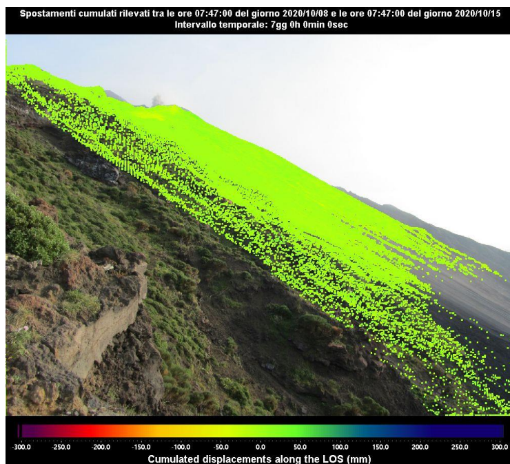
Figura 1 - Mappa degli spostamenti cumulati registrati dal sistema GB-InSAR NE190 riferito al tempo di 7 giorni, dalle ore 07:47 UTC (09:47 ore locali) del 08 ottobre 2020 alle ore 07:47 UTC (09:47 ore locali) del 15 ottobre 2020.
