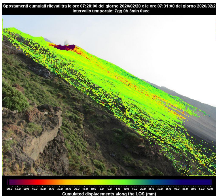
Figura 1 - Mappa degli spostamenti cumulati registrati dal sistema GB-InSAR NE190 riferito al tempo di 7 giorni e 3 minuti, dalle ore 07:28 UTC (08:28 ore locali) del 20 febbraio 2020 alle ore 07:31 UTC (08:31 ore locali) del 27 febbraio 2020.
