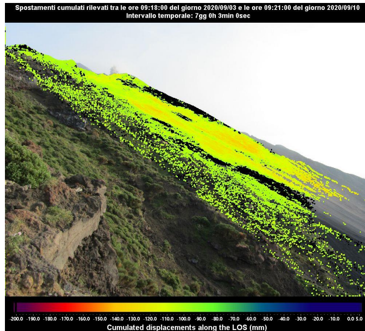
Figura 1 - Mappa degli spostamenti cumulati registrati dal sistema GB-InSAR NE190 riferito al tempo di 7 giorni e 3 minuti, dalle ore 09:10 UTC (11:10 ore locali) del 03 settembre 2020 alle ore 09:21 UTC (11:21 ore locali) del 10 settembre 2020.
