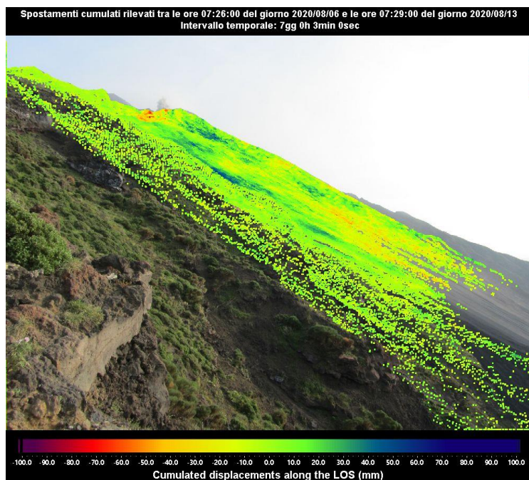
Figura 3 - Mappa degli spostamenti cumulati registrati dal sistema GB-InSAR NE190 riferito al tempo di 7 giorni e 3 minuti, dalle ore 07:26 UTC (09:26 ore locali) del 06 agosto 2020 alle ore 07:29 UTC (09:29 ore locali) del 13 agosto 2020.
