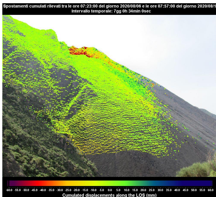
Figura 1 - Mappa degli spostamenti cumulati registrati dal sistema GB-InSAR NE400 riferito al tempo di 7 giorni e 34 minuti, dalle ore 07:23 UTC (09:23 ore locali) del 06 agosto 2020 alle ore 07:57 UTC (09:57 ore locali) del 13 agosto 2020.
