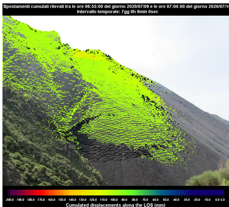
Figura 2 - Mappa degli spostamenti cumulati registrati dal sistema GB-InSAR NE400 riferito al tempo di 7 giorni e 9 minuti, dalle ore 06:55 UTC (08:55 ore locali) del 9 luglio 2020 alle ore 07:04 UTC (09:04 ore locali) del 16 luglio 2020.
