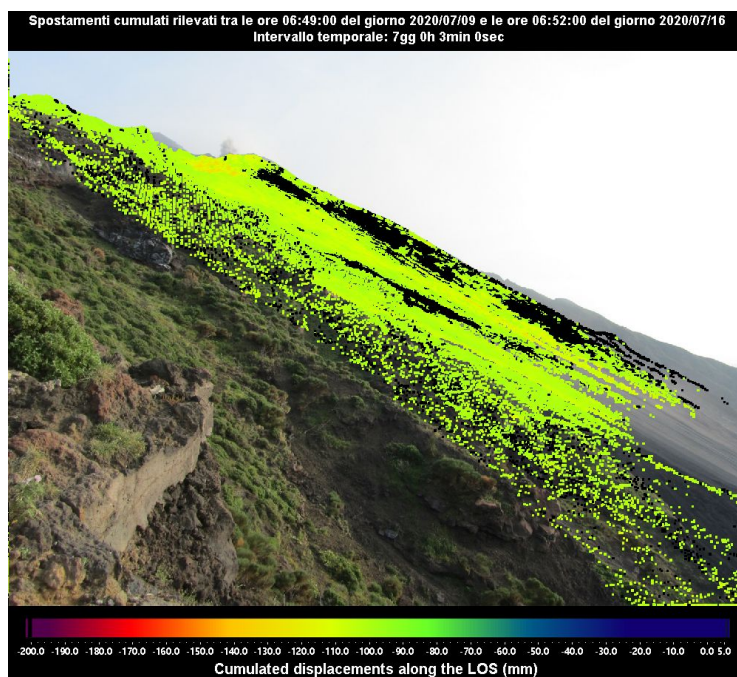
Figura 3 - Mappa degli spostamenti cumulati registrati dal sistema GB-InSAR NE190 riferito al tempo di 7 giorni e 3 minuti, dalle ore 06:49 UTC (08:49 ore locali) del 9 luglio 2020 alle ore 06:52 UTC (08:52 ore locali) del 16 luglio 2020.
