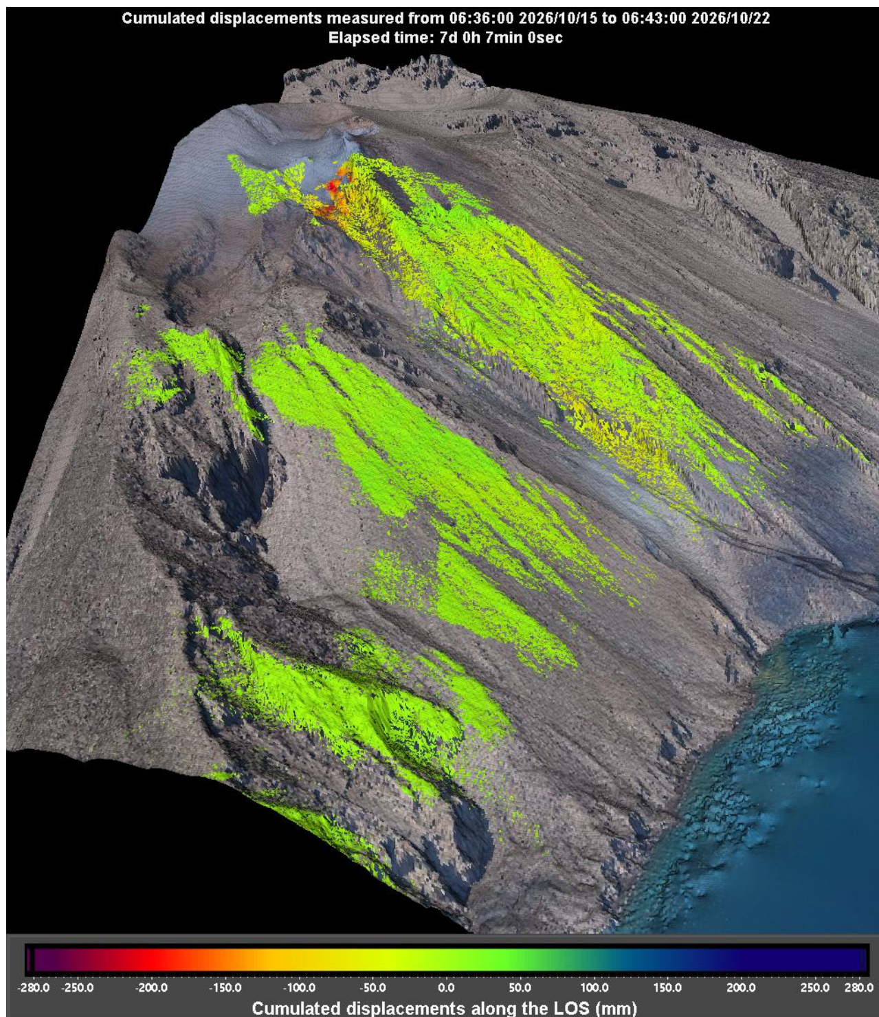
Figura 2 - Mappa cumulata degli spostamenti registrata dal sistema GBInSAR NE190 riferito al tempo di 7 giorni e 7 minuti dalle ore 06:36 UTC (08:36 ora locale) del 15 ottobre 2026 alle ore 06:34 UTC (08:34 ora locale) del 22 ottobre 2026.
