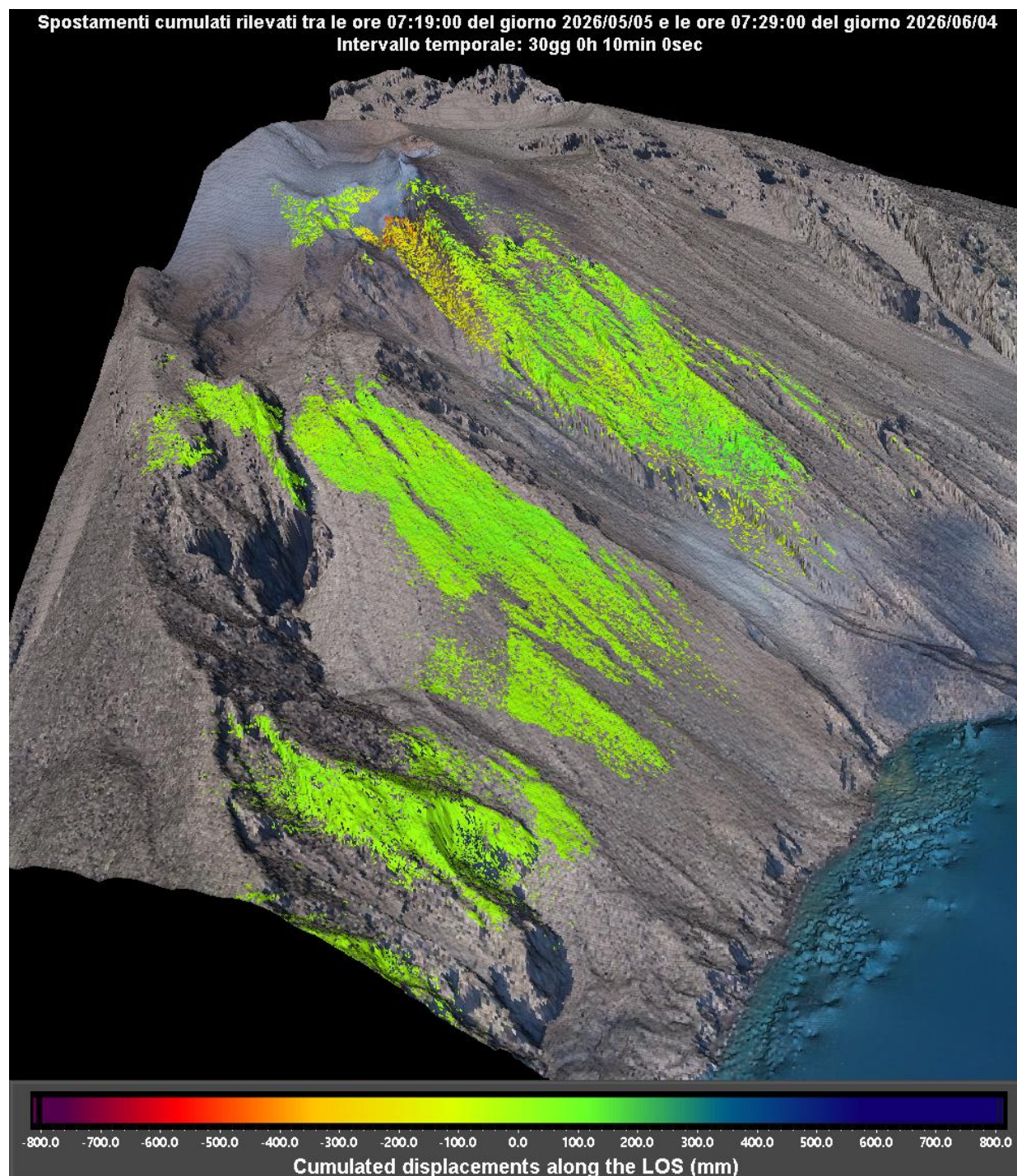
Figura 2 - Mappa cumulata degli spostamenti registrata dal sistema GBInSAR NE190 riferito al tempo di 30 giorni e 10 minuti dalle ore 07:19 UTC (08:19 ora locale) del 05 maggio 2026 alle ore 07:29 UTC (08:29 ora locale) del 04 giugno 2026.
