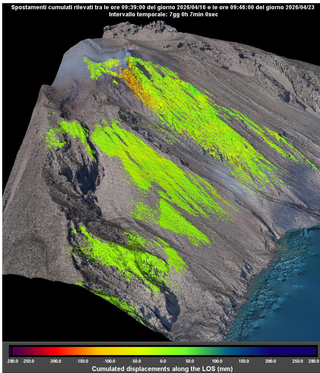
Figura 2 - Mappa cumulata degli spostamenti registrata dal sistema GBInSAR NE190 riferito al tempo di 7 giorni e 7 minuto dalle ore 09:39 UTC (11:39 ora locale) del 16 aprile 2026 alle ore 09:46 UTC (11:46 ora locale) del 23 aprile 2026.
