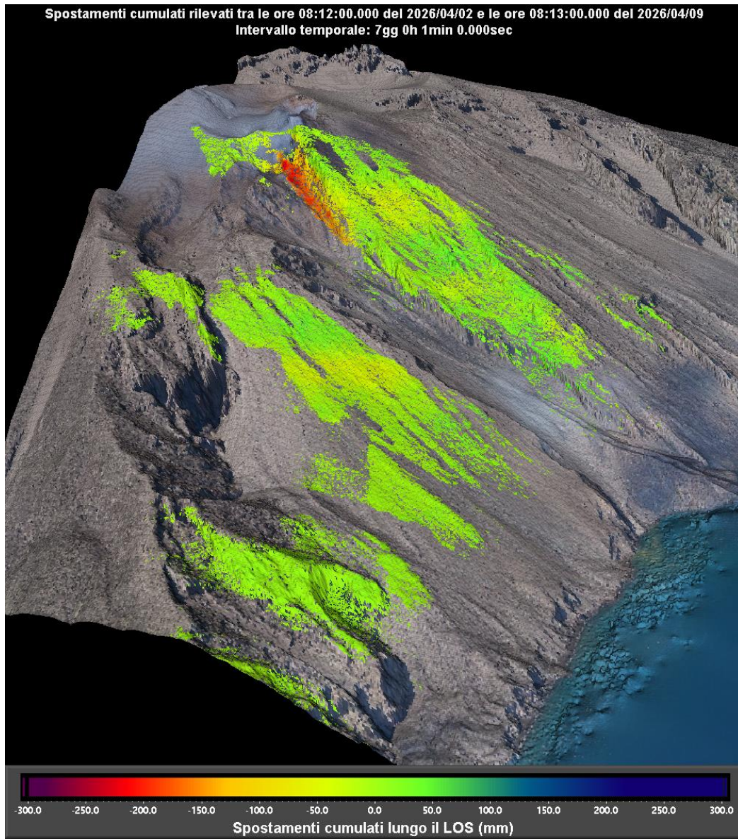
Figura 2 - Mappa cumulata degli spostamenti registrata dal sistema GBInSAR NE190 riferito al tempo di 7 giorni e 1 minuto dalle ore 08:12 UTC (10:12 ora locale) del 02 aprile 2026 alle ore 08:13 UTC (10:13 ora locale) del 09 aprile 2026.
