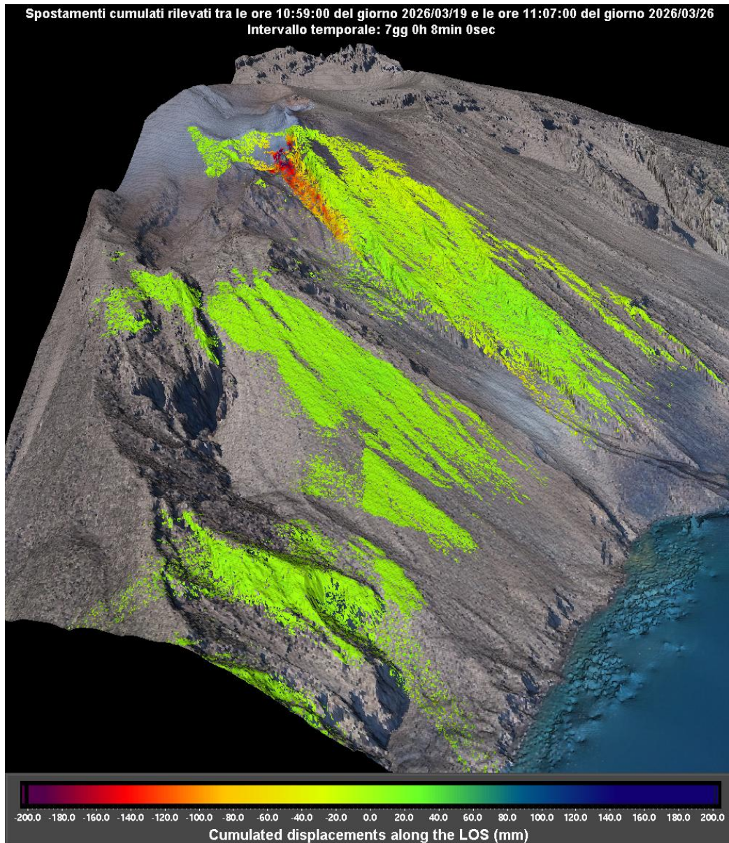
Figura 1 - Mappa cumulata degli spostamenti registrata dal sistema GBInSAR NE190 riferito al tempo di 7 giorni e 8 minuti dalle ore 10:59 UTC (11:59 ora locale) del 19 marzo 2026 alle ore 11:07 UTC (12:07 ora locale) del 26 marzo 2026.
