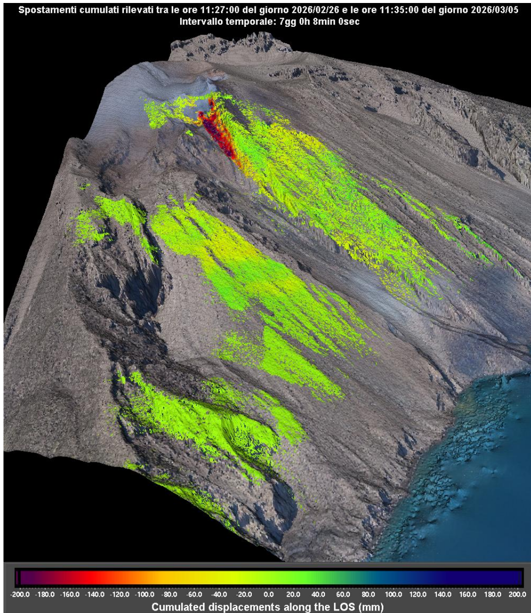
Figura 1 - Mappa cumulata degli spostamenti registrata dal sistema GBInSAR NE190 riferito al tempo di 7 giorni e 8 minuti dalle ore 11:27 UTC (12:27 ora locale) del 26 febbraio 2026 alle ore 11:35 UTC (12:35 ora locale) del 05 marzo 2026.
