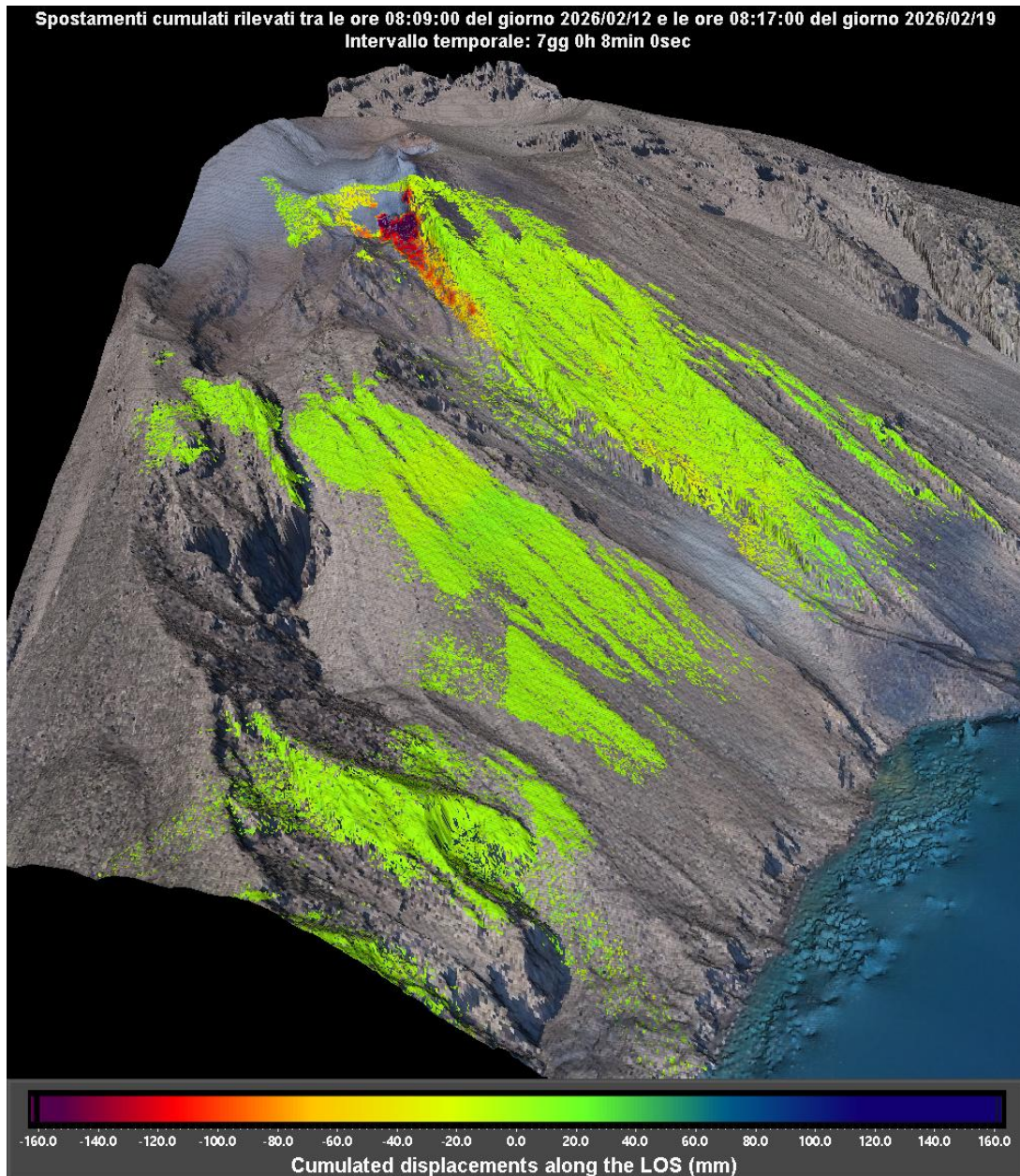
Figura 1 - Mappa cumulata degli spostamenti registrata dal sistema GBInSAR NE190 riferito al tempo di 7 giorni e 8 minuti dalle ore 08:09 UTC (09:09 ora locale) del 12 febbraio 2026 alle ore 08:17 UTC (09:17 ora locale) del 19 febbraio 2026.
