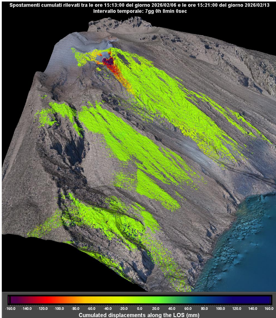
Figura 1 - Mappa cumulata degli spostamenti registrata dal sistema GBInSAR NE190 riferito al tempo di 7 giorni e 8 minuti dalle ore 15:30 UTC (16:30 ora locale) del 06 febbraio 2026 alle ore 15:21 UTC (16:21 ora locale) del 13 gennaio 2026.
