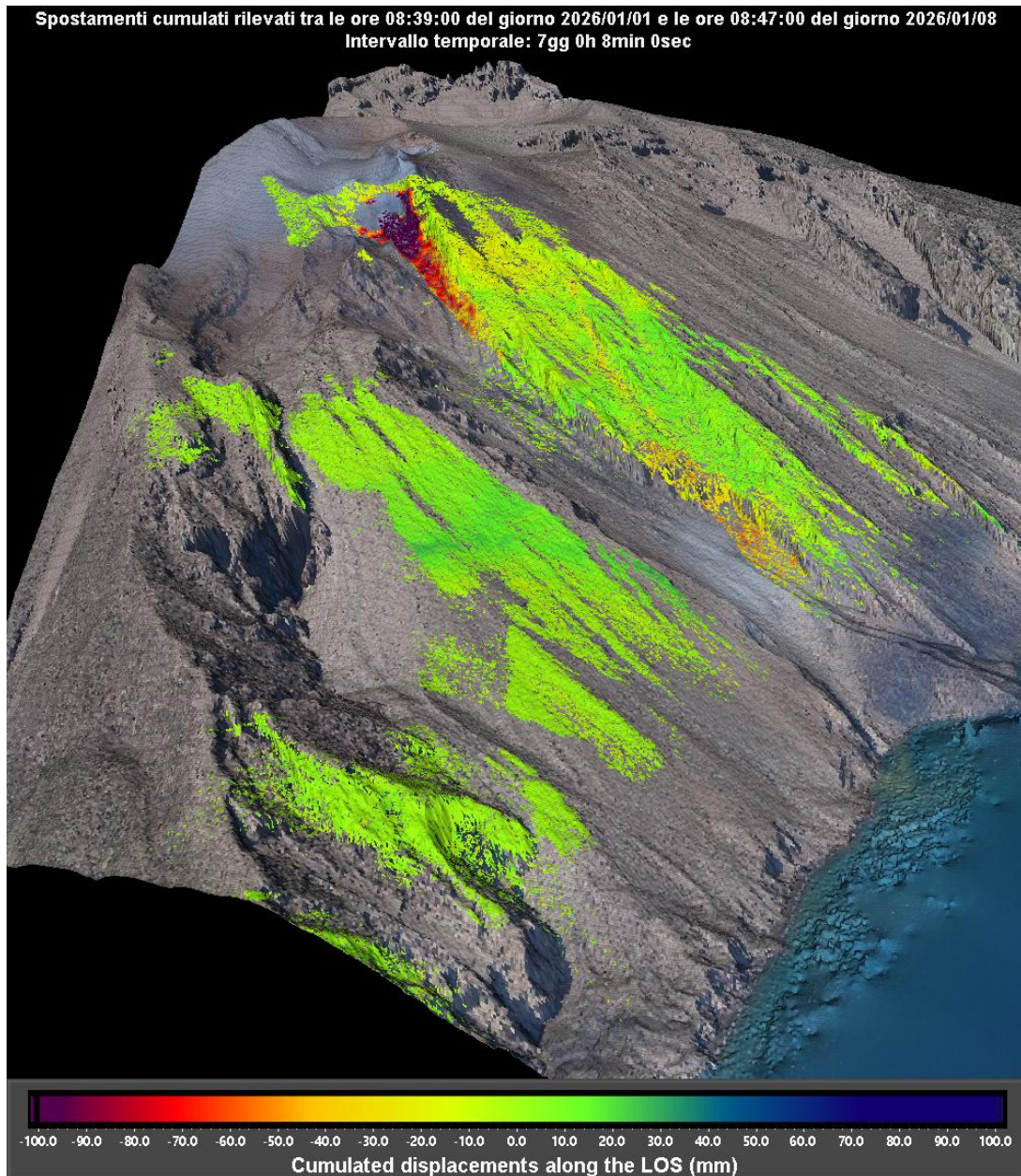
Figura 1 - Mappa cumulata degli spostamenti registrata dal sistema GBInSAR NE190 riferito al tempo di 7 giorni e 8 minuti dalle ore 08:39 UTC (09:39 ora locale) del 01 gennaio 2026 alle ore 08:47 UTC (09:47 ora locale) del 08 gennaio 2026.
