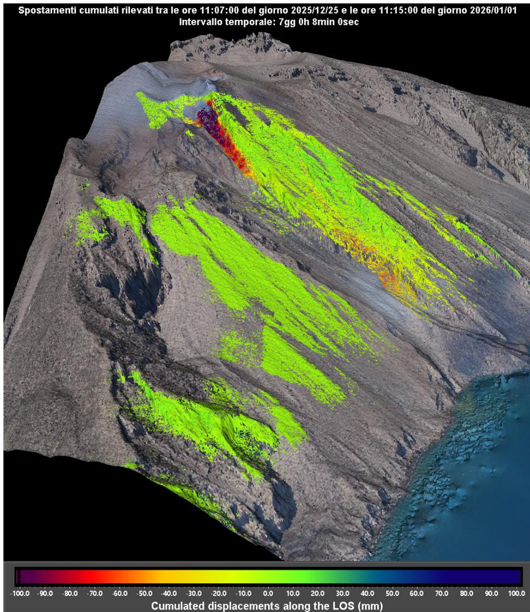
Figura 1 - Mappa cumulata degli spostamenti registrata dal sistema GBInSAR NE190 riferito al tempo di 7 giorni e 8 minuti dalle ore 11:07 UTC (12:07 ora locale) del 25 dicembre 2025 alle ore 11:15 UTC (12:15 ora locale) del 01 gennaio 2026.
