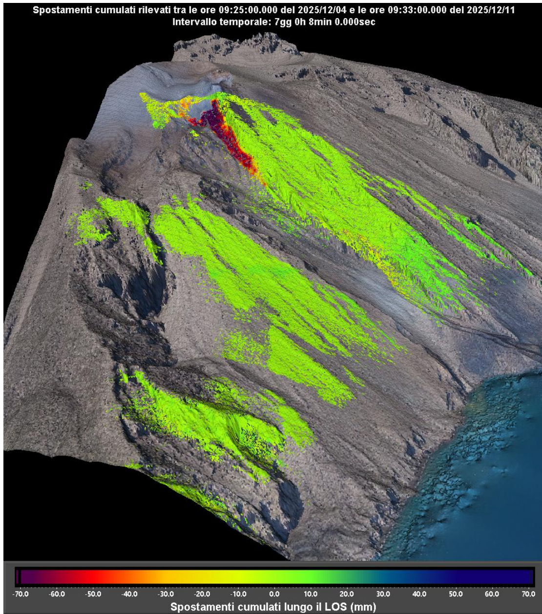
Figura 1 - Mappa cumulata degli spostamenti registrata dal sistema GBInSAR NE190 riferito al tempo di 7 giorni e 8 minuti dalle ore 09:25 UTC (10:25 ora locale) del 04 dicembre 2025 alle ore 09:33 UTC (10:33 ora locale) del 11 dicembre 2025.
