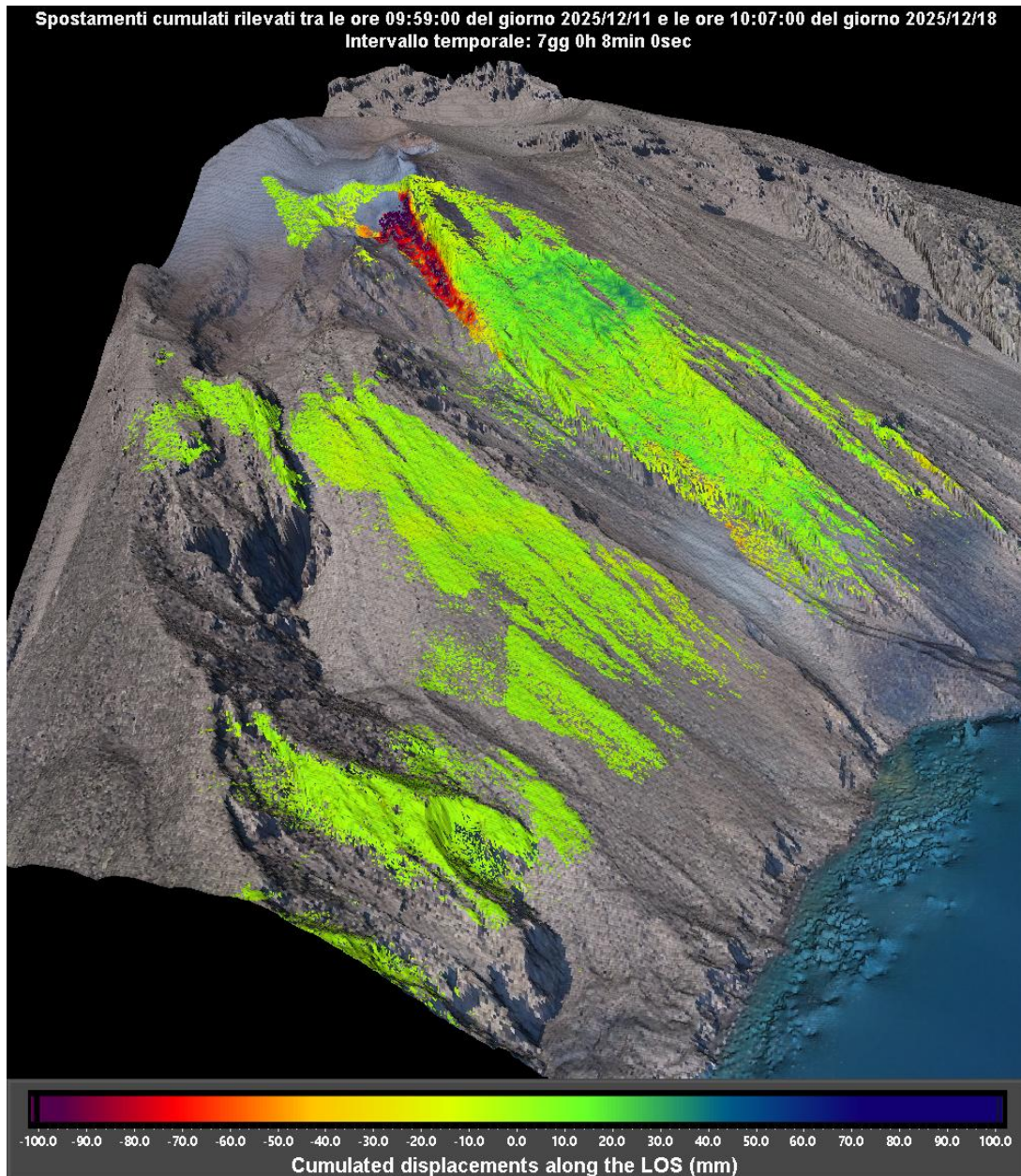
Figura 1 - Mappa cumulata degli spostamenti registrata dal sistema GBInSAR NE190 riferito al tempo di 7 giorni e 8 minuti dalle ore 09:59 UTC (10:59 ora locale) del 11 dicembre 2025 alle ore 10:07 UTC (11:07 ora locale) del 18 dicembre 2025.
