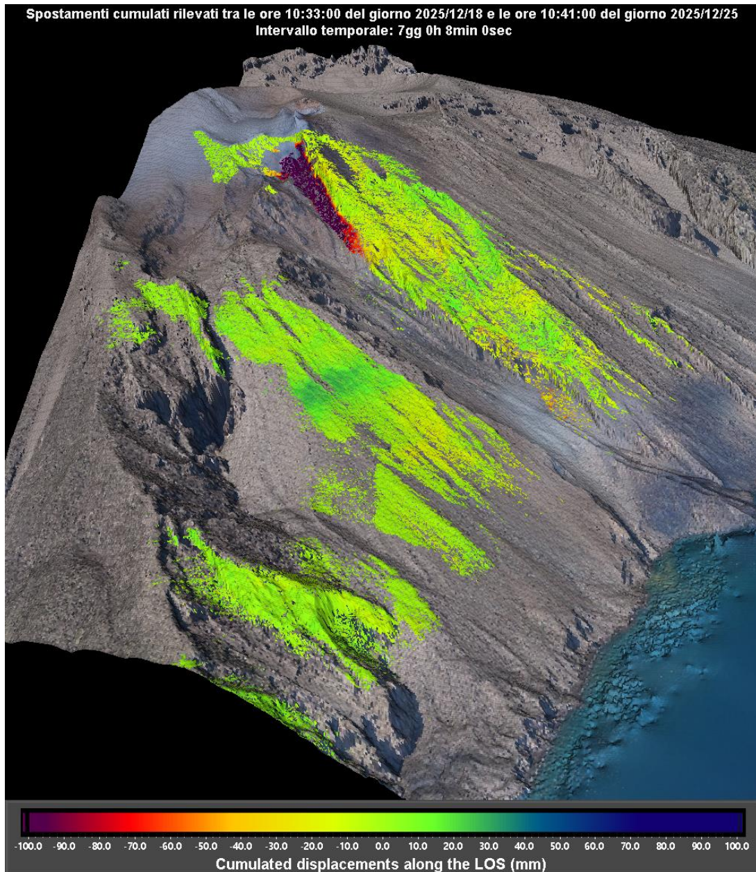
Figura 1 - Mappa cumulata degli spostamenti registrata dal sistema GBInSAR NE190 riferito al tempo di 7 giorni e 8 minuti dalle ore 10:33 UTC (11:33 ora locale) del 18 dicembre 2025 alle ore 10:41 UTC (11:41 ora locale) del 25 dicembre 2025.
