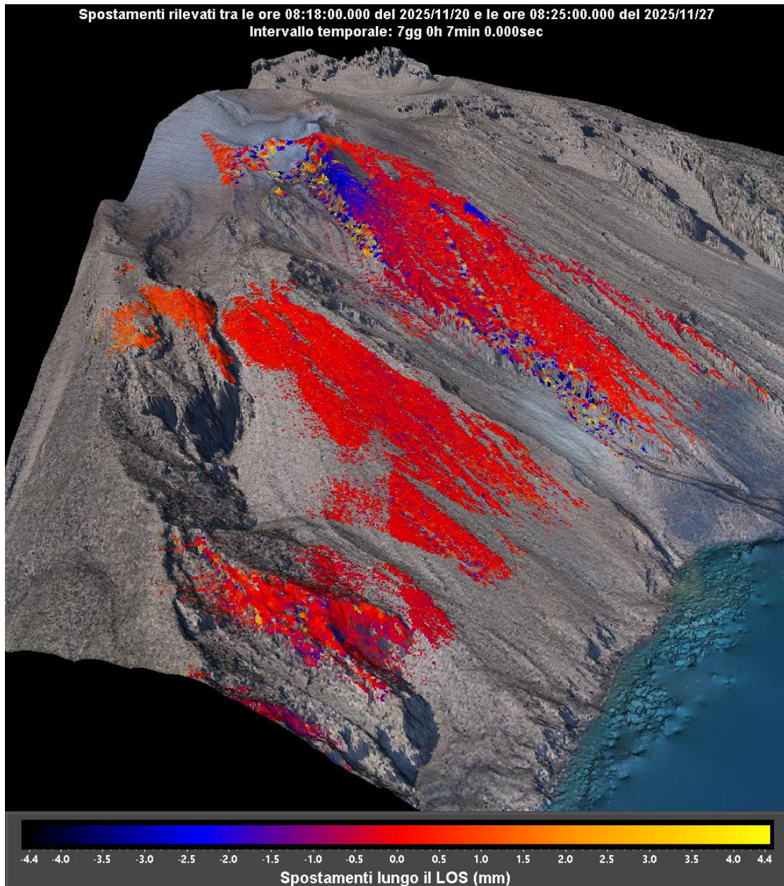
Figura 1 - Interferogramma registrato dal sistema GBInSAR NE190 riferito al tempo di 7 giorni e 7 minuti dalle ore 08:18 UTC (09:18 ora locale) del 20 novembre 2025 alle ore 08:25 UTC (09:25 ora locale) del 27 novembre 2025.
