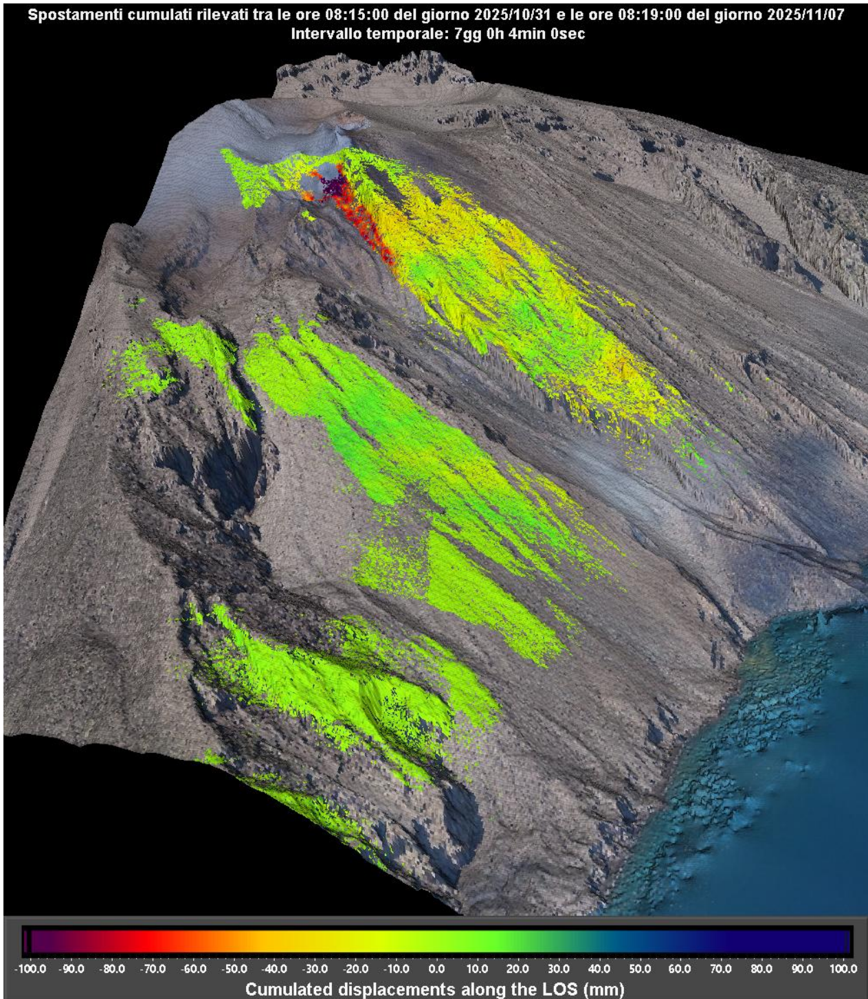
Figura 2 - Mappa cumulata degli spostamenti registrata dal sistema GBInSAR NE190 riferito al tempo di 7 giorni e 4 minuti dalle ore 08:15 UTC (10:15 ora locale) del 31 ottobre 2025 alle ore 08:19 UTC (09:19 ora locale) del 07 novembre 2025.
