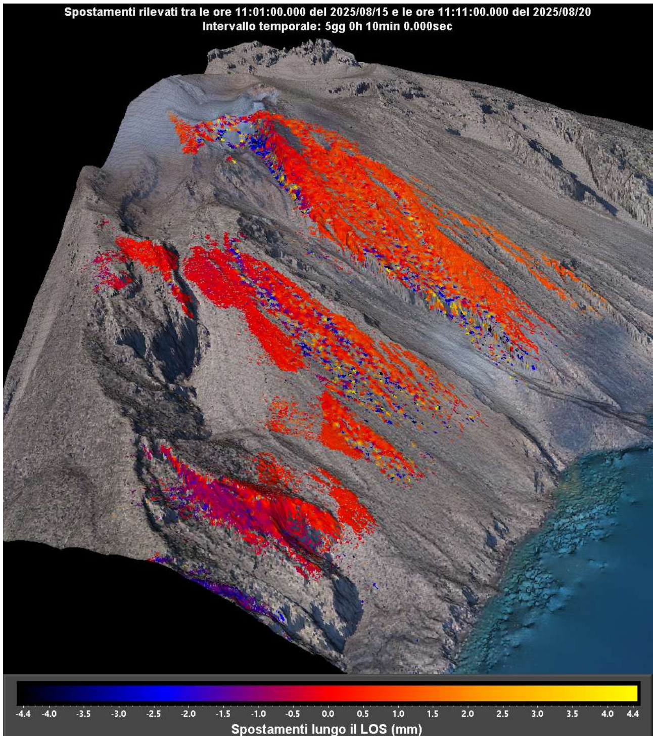
Figura 2 – Mappa cumulata delle deformazioni registrata dal sistema GBInSAR NE190 riferito al tempo di 5 giorni e 10 minuti dalle ore 11:01 UTC (13:01 ora locale) del 15 agosto 2024 alle ore 11:11 UTC (13:11 ora locale) del 20 agosto 2025.
