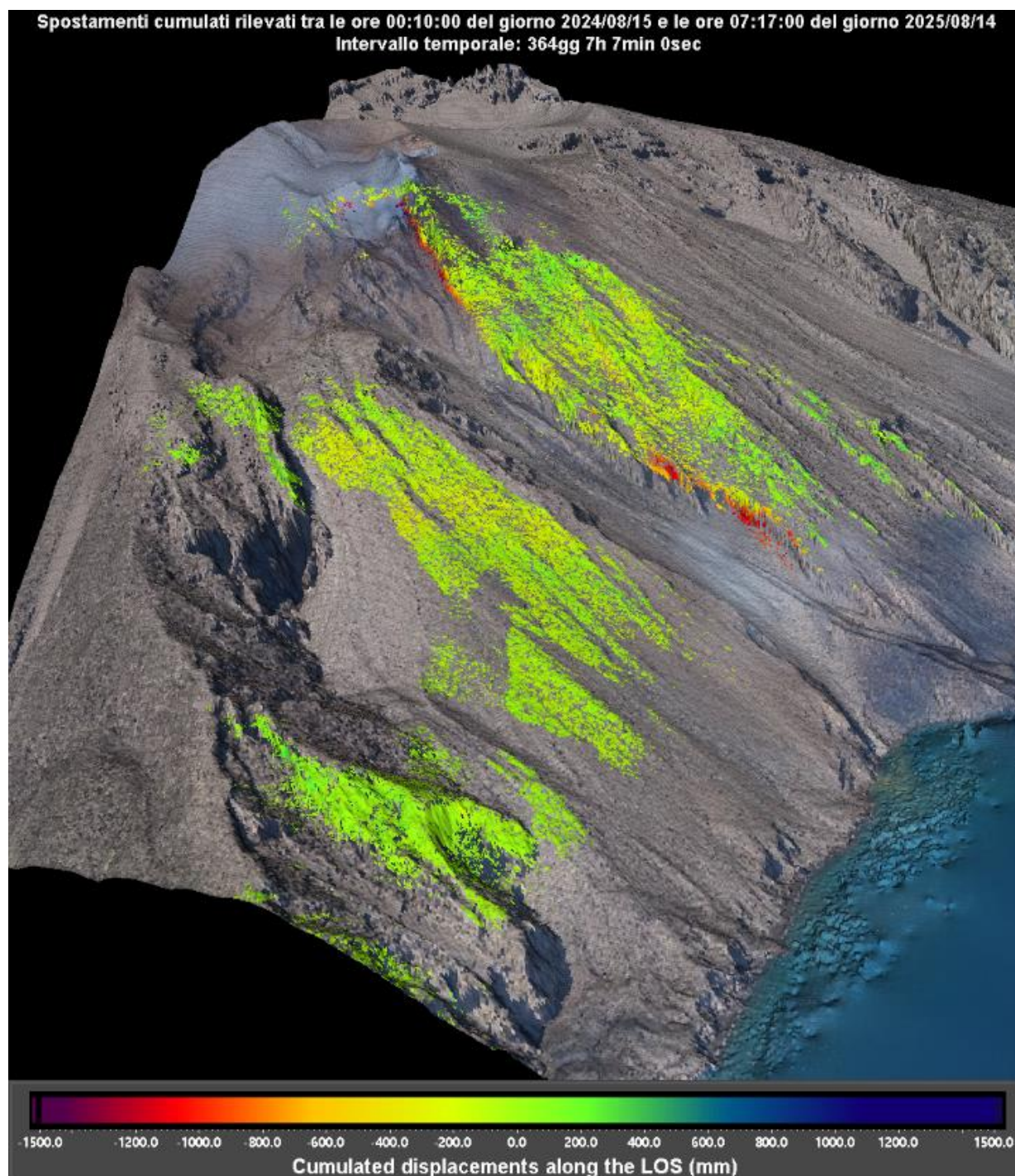
Figura 2 – Mappa cumulata delle deformazioni registrata dal sistema GBInSAR NE190 riferito al tempo di 364 giorni 7 ore 7 minuti dalle ore 00:10 UTC (02:10 ora locale) del 15 agosto 2024 alle ore 07:17 UTC (09:17 ora locale) del 14 agosto 2025.
