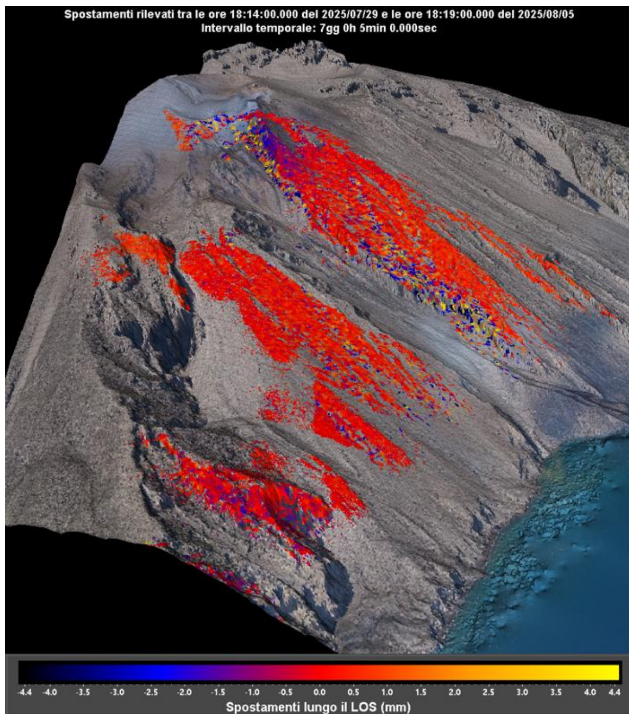
Figura 2 – Interferogramma registrato dal sistema GBInSAR NE190 riferito al tempo di 7 giorni e 5 minuti dalle ore 18:14 UTC (20:14 ora locale) del 29 luglio 2025 alle ore 18:19 UTC (20:19 ora locale) del 5 agosto 2025.
