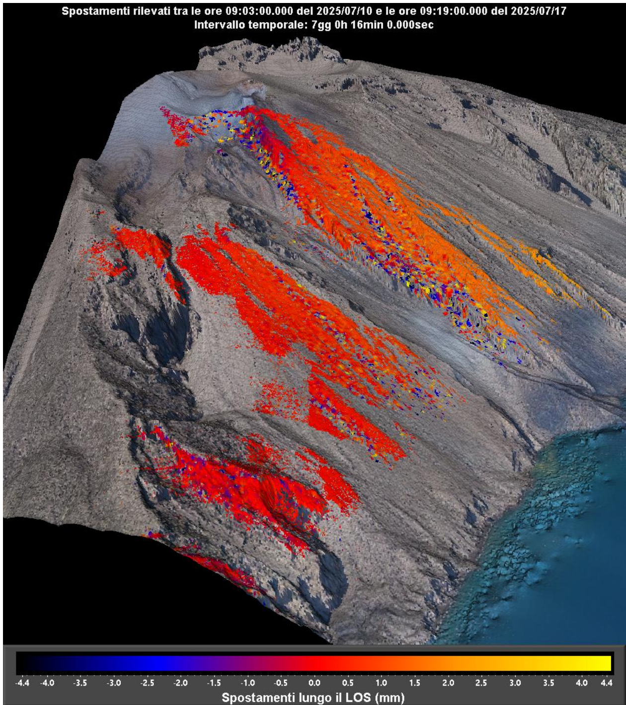
Figura 2 – Mappa cumulata delle deformazioni registrata dal sistema GBInSAR NE190 riferito al tempo di 7 giorni 16 minuti dalle ore 09:03 UTC (11:03 ora locale) del 10 luglio 2024 alle ore 09:19 UTC (11:19 ora locale) del 17 luglio 2025.
