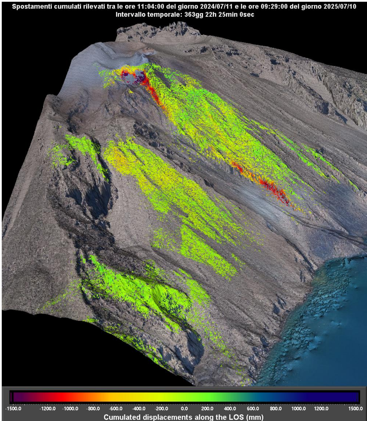
Figura 2 – Mappa cumulata delle deformazioni registrata dal sistema GBInSAR NE190 riferito al tempo di 353 giorni 22 ore e 25 minuti dalle ore 11:04 UTC (01:04 ora locale) del 11 luglio 2024 alle ore 09:29 UTC (10:29 ora locale) del 10 luglio 2025.
