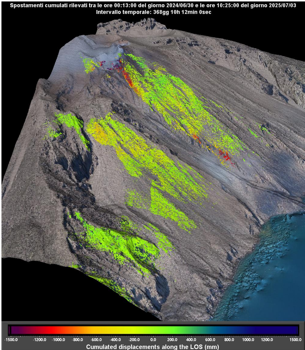
Figura 2 – mappa cumulata delle deformazioni registrata dal sistema GBInSAR NE190 riferito al tempo di 368 giorni 10 ore e 12 minuti dalle ore 00:13 UTC (01:13 ora locale) del 30 giugno 2024 alle ore 10:25 UTC (11:25 ora locale) del 03 luglio 2025.
