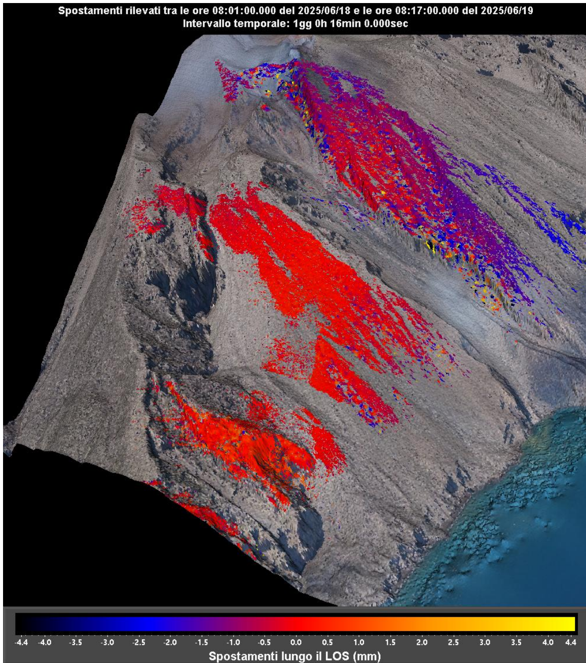
Figura 2 - Interferogramma registrato dal sistema GBInSAR NE190 riferito al tempo di 1 giorno e 16 minuti dalle ore 08:01 UTC (09:01 ora locale) del 18 giugno 2025 alle ore 08:17 UTC (09:17 ora locale) del 19 giugno 2025.
