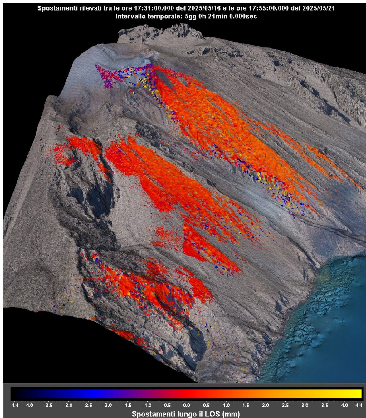
Figura 2 – Interferogramma registrato dal sistema GBInSAR NE190 riferito al tempo di 5 giorni e 24 minuti dalle ore 17:31 UTC (19:31 ora locale) del 16 maggio 2025 alle ore 17:55 UTC (19:55 ora locale) del 21 maggio 2025.
