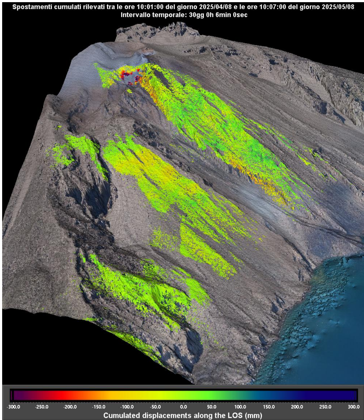
Figura 2 – Mappa cumulata delle deformazioni registrata dal sistema GBInSAR NE190 riferito al tempo di 30 giorni e 6 minuti dalle ore 10:01 UTC (12:01 ora locale) dell'8 aprile 2025 alle ore 10:07 UTC (12:07 ora locale) del 08 maggio 2025.
