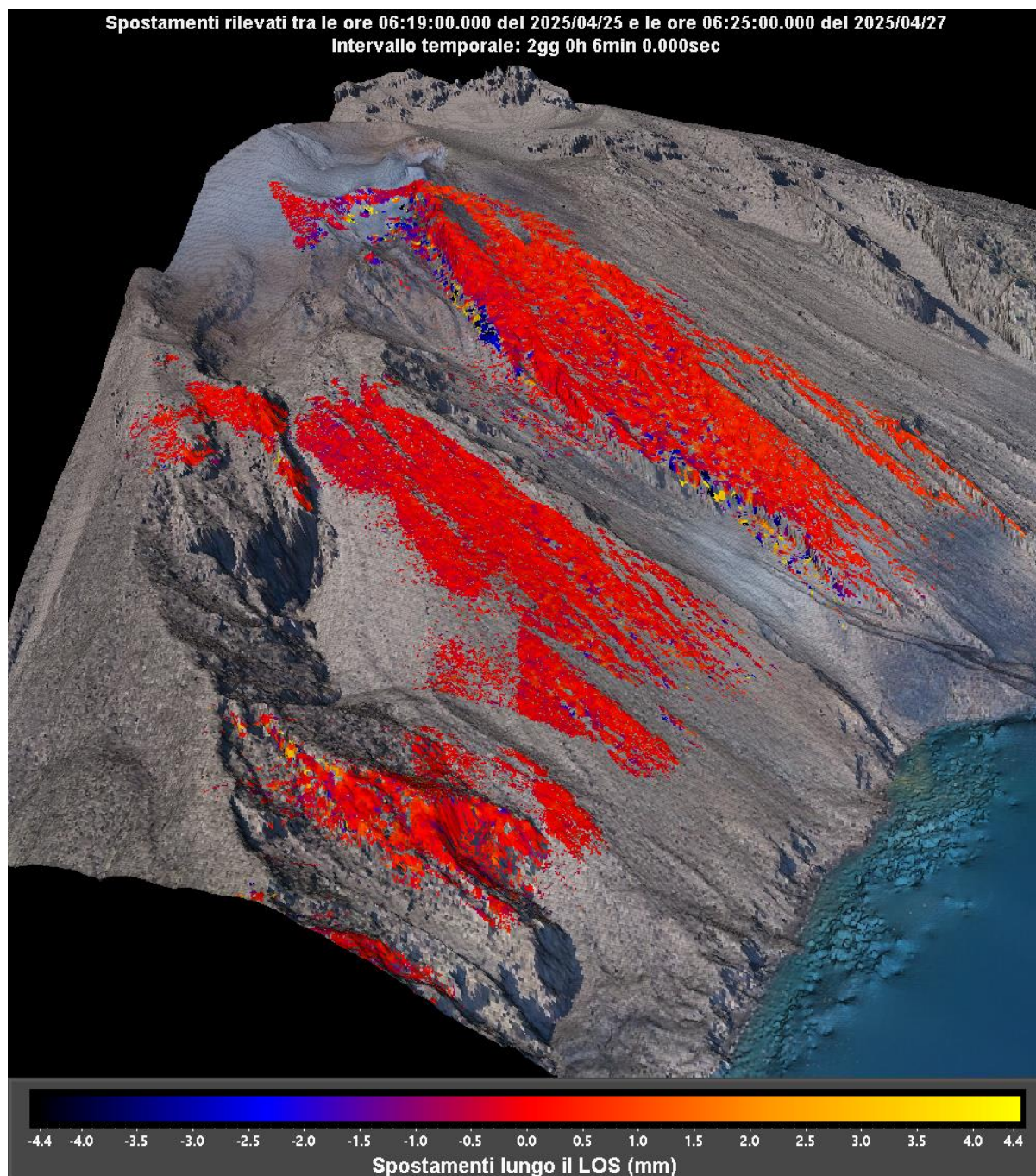
Figura 2 – Interferogramma registrato dal sistema GBInSAR NE190 riferito al tempo di 2 giorni e 6 minuti dalle ore 06:19 UTC (07:19 ora locale) del 25 aprile 2025 alle ore 06:25 UTC (07:25 ora locale) del 27 aprile 2025.
