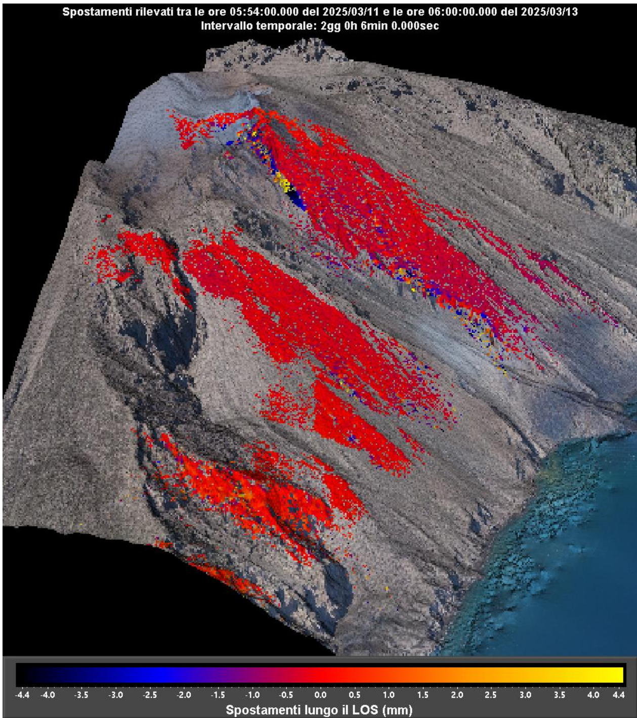
Figura 2 - Interferogramma registrato dal sistema GBInSAR NE190 riferito al tempo di 2 giorni e 6 minuti dalle ore 05:54 UTC (06:54 ora locale) del 11 marzo 2025 alle ore 06:00 UTC (07:00 ora locale) del 13 marzo 2025.
