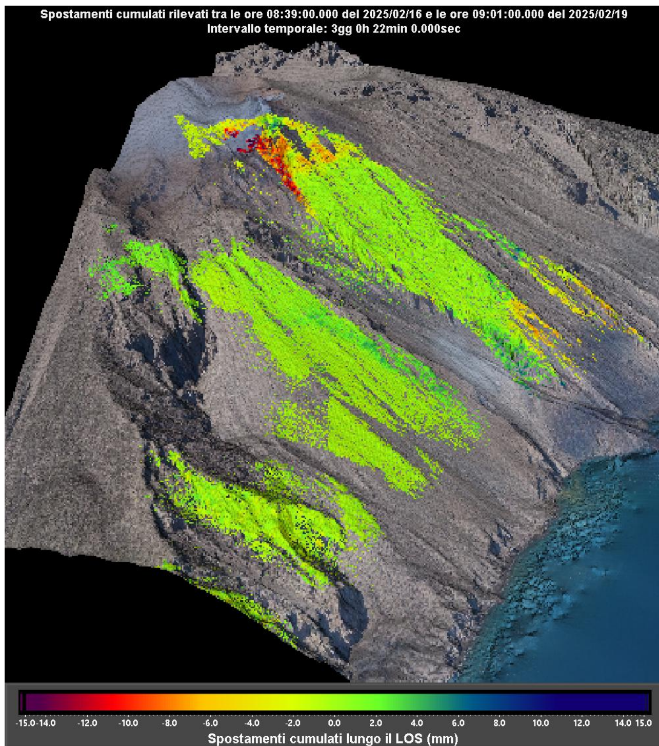
Figura 2 – mappa cumulata delle deformazioni registrata dal sistema GBInSAR NE190 riferito al tempo di 3 giorni e 22 minuti dalle ore 08:39 UTC (09:39 ora locale) del 16 febbraio 2025 alle ore 09:01 UTC (10:01 ora locale) del 19 febbraio 2025.
